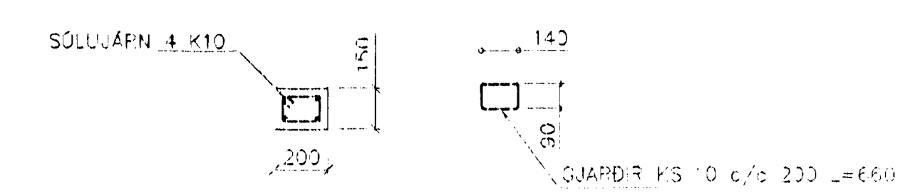
SÚLA S1 1:20
