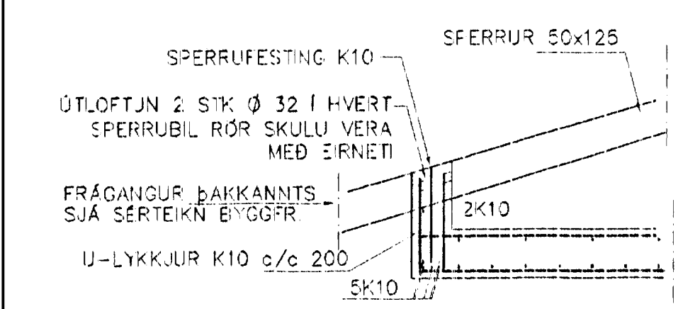
SNÍÐ 6 1:20
