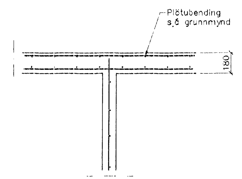
SNÍÐ 5 1:20
