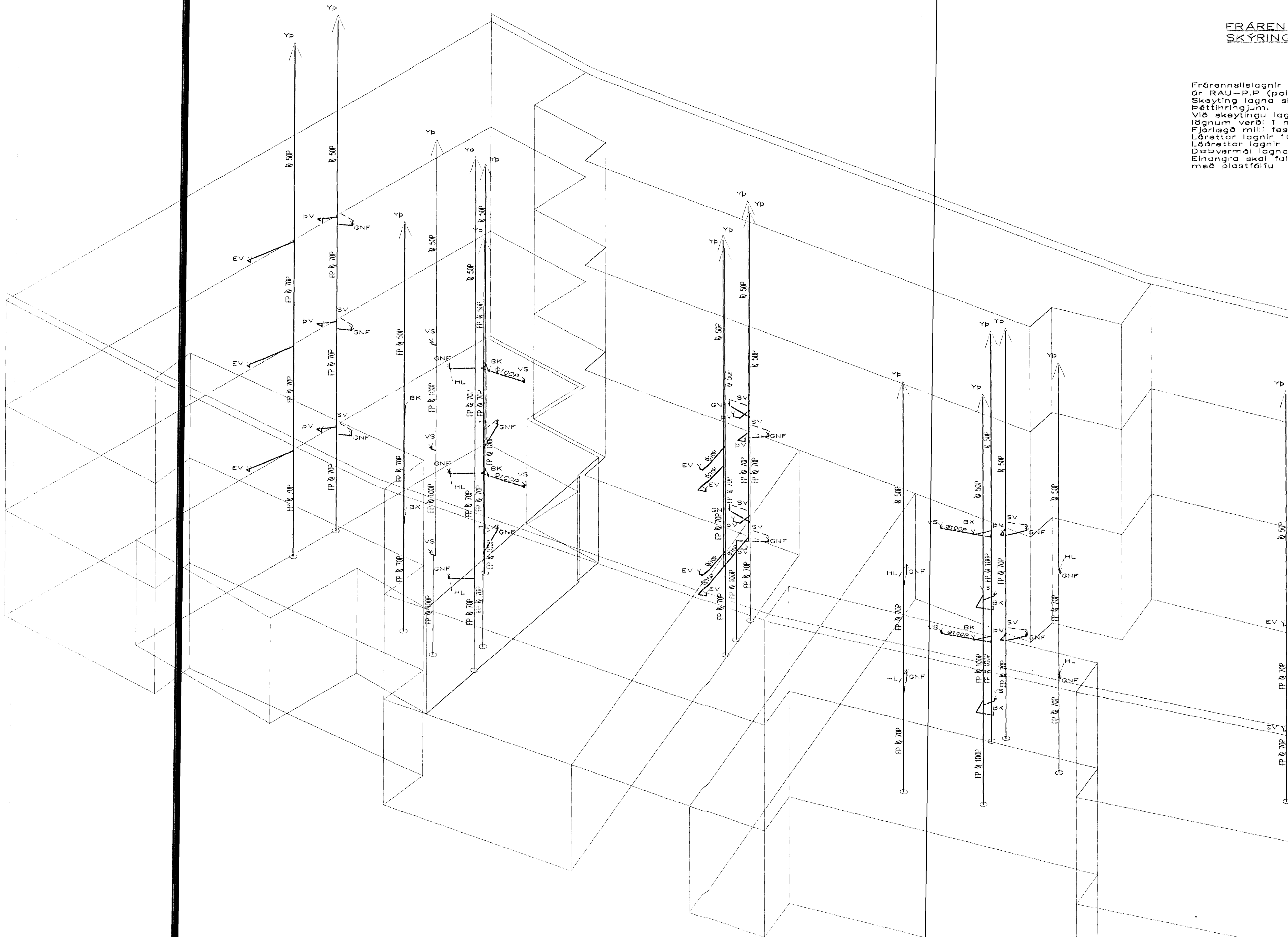
RÖMMYND FRÆRENNSLISLAGNA 1:50
