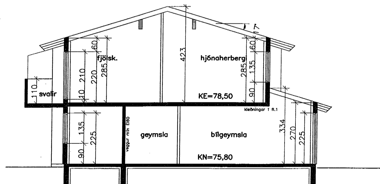
skurður B-B
