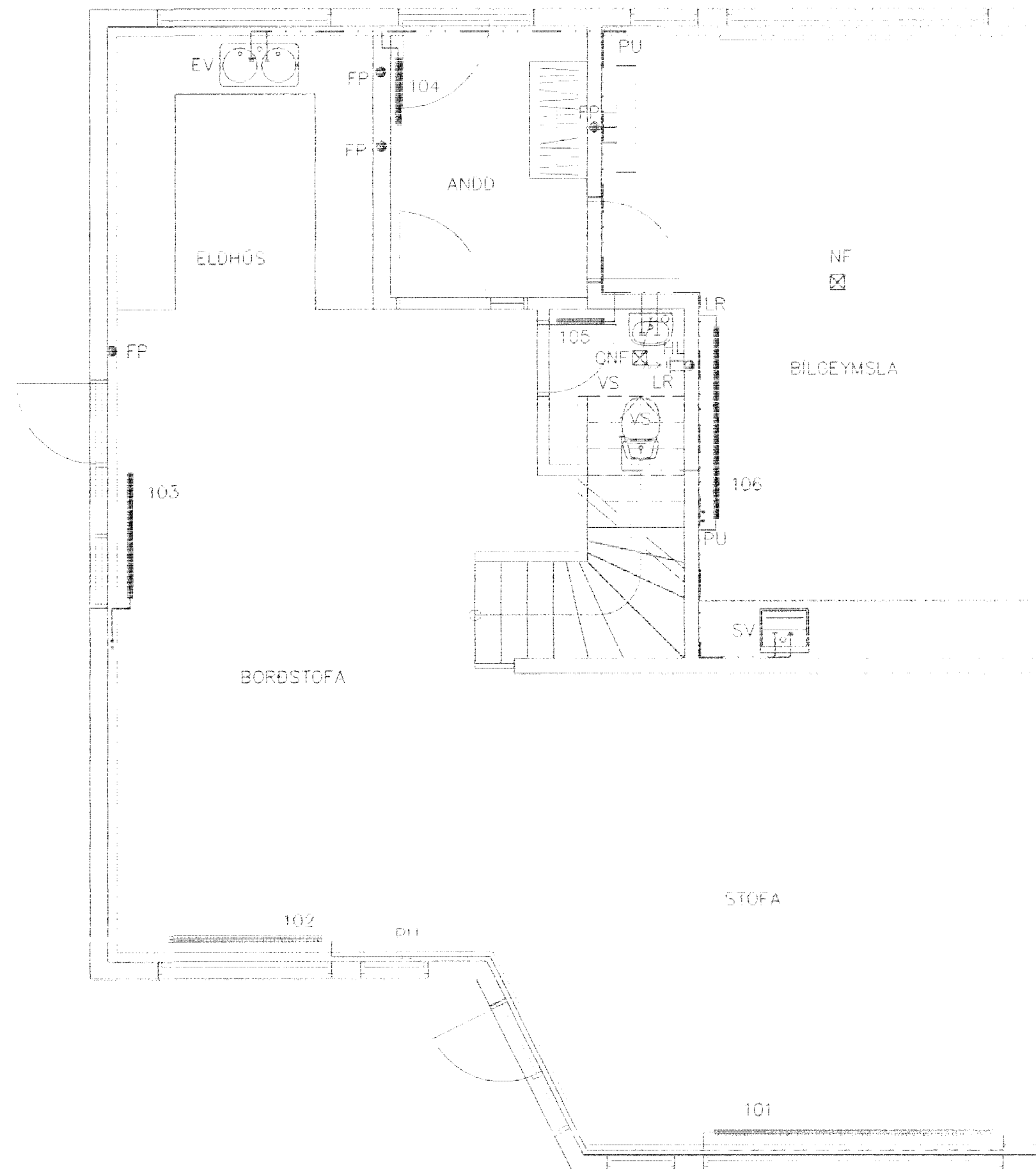
GRUNNMYND 1 HÆÐ 1:50
