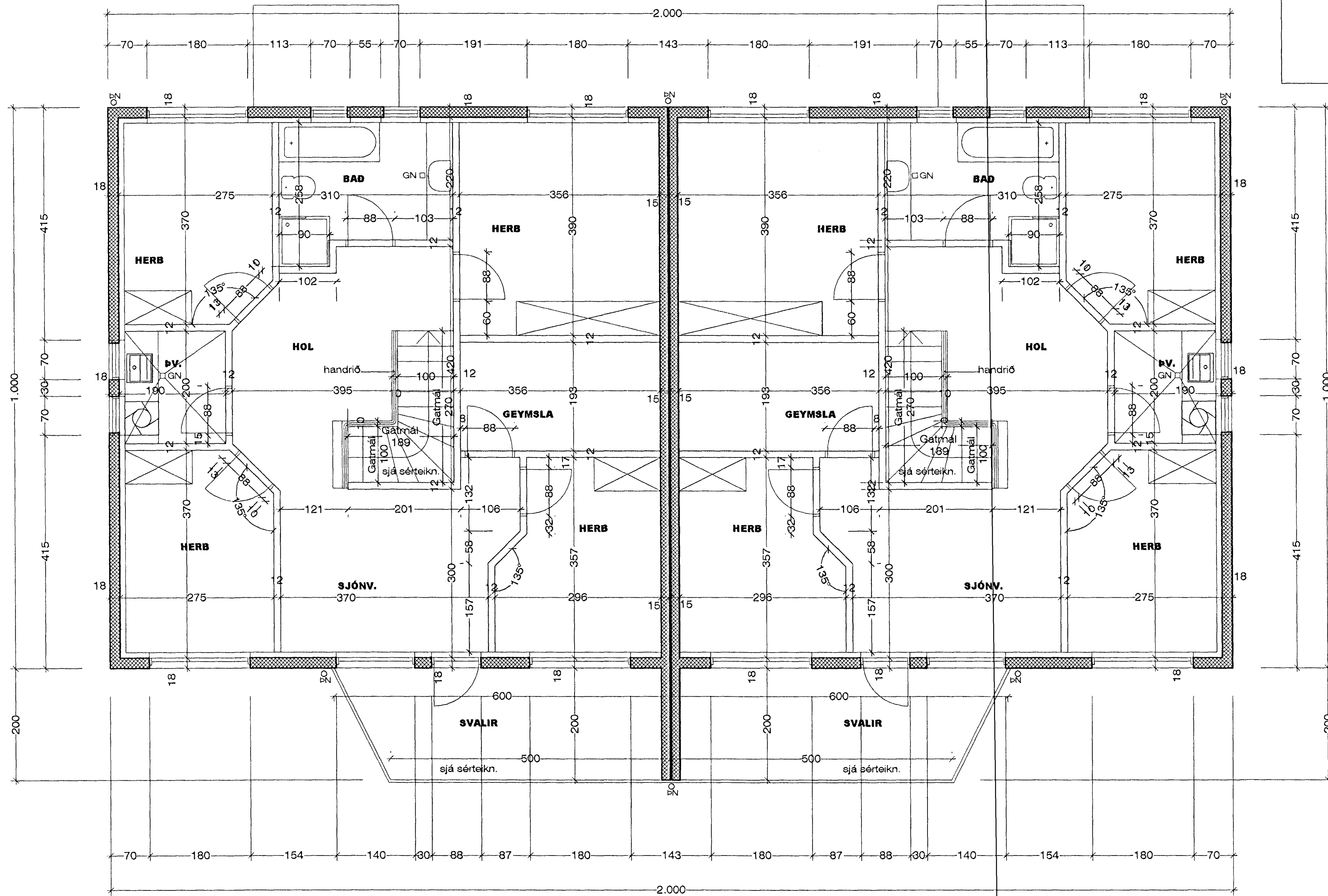
Grunnmynd 2. hæð
