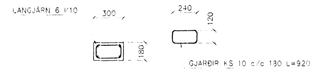
SÓLA S2 1:20
