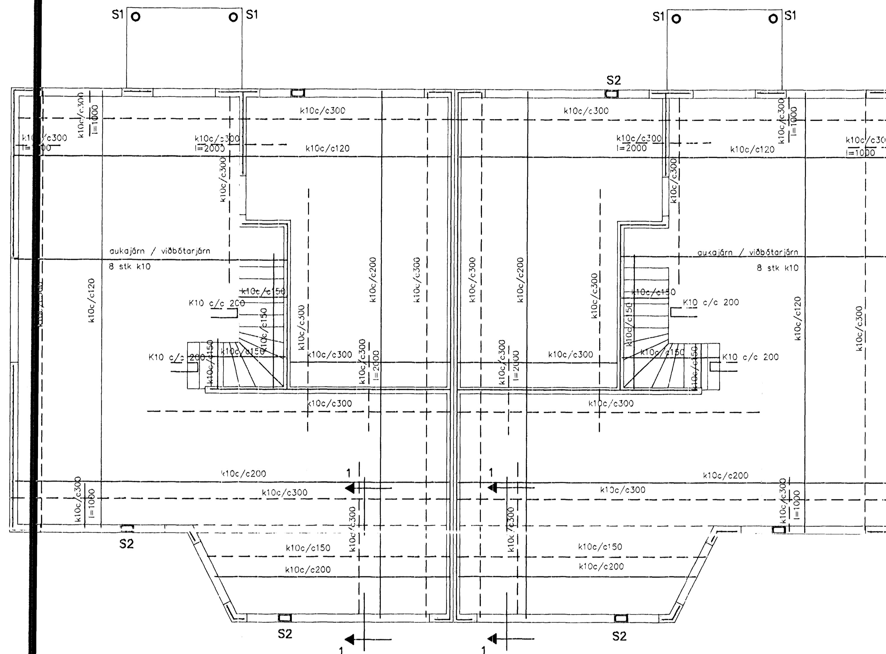
GRUNNMYND 1:50
