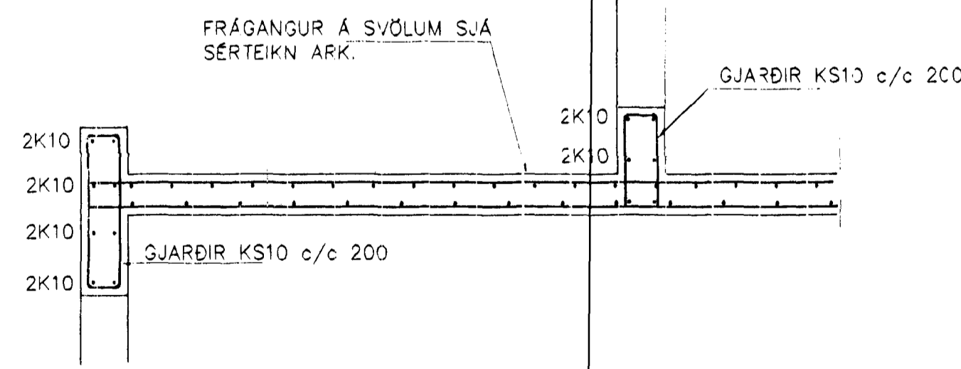
SNÍÐ 1-1 1:20
