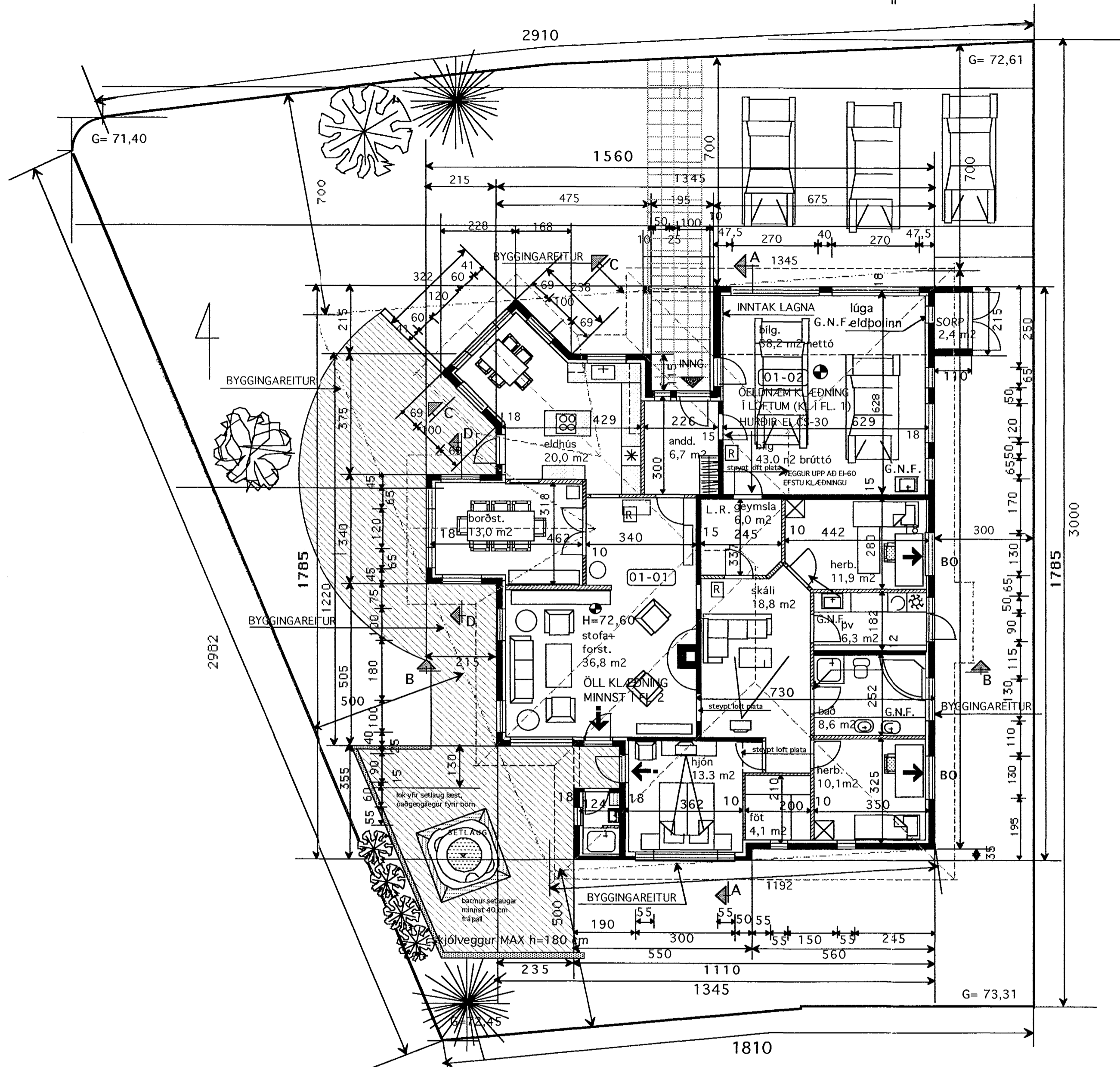
GRUNNMYND 1 :100 Nánari málsetning sjá tekn. V-1
