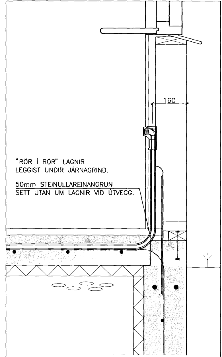
STADSETNING LAGNA Mkv. 1:10
