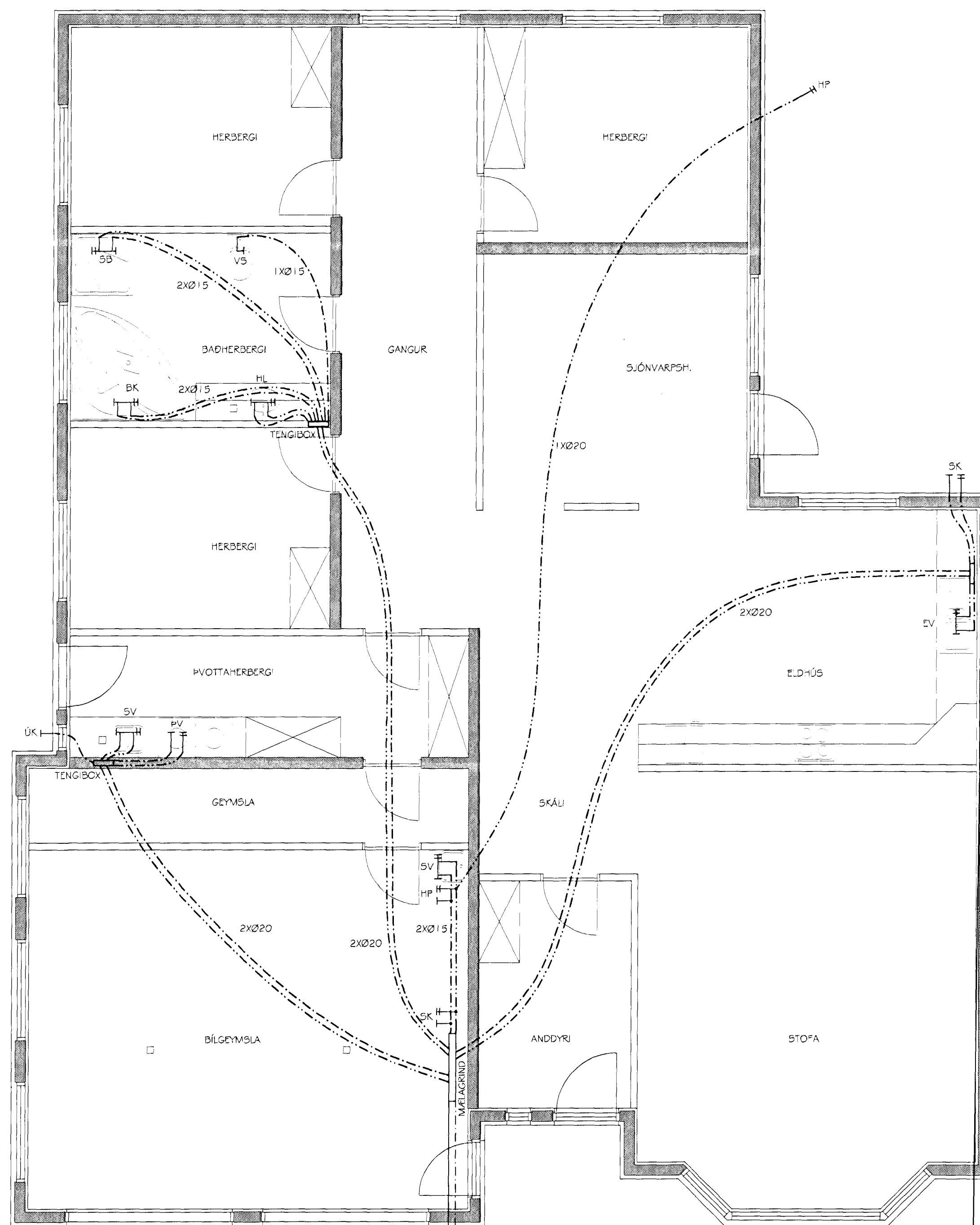
NEYSLUVATNSLAGNIR GRUNNMYND MKV. 1:50
