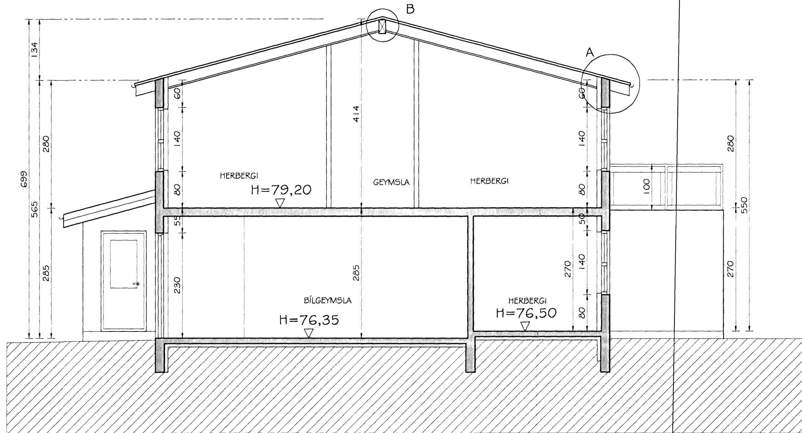
SVÖLUÁS 3 SNID A-A MKV. 1:50
