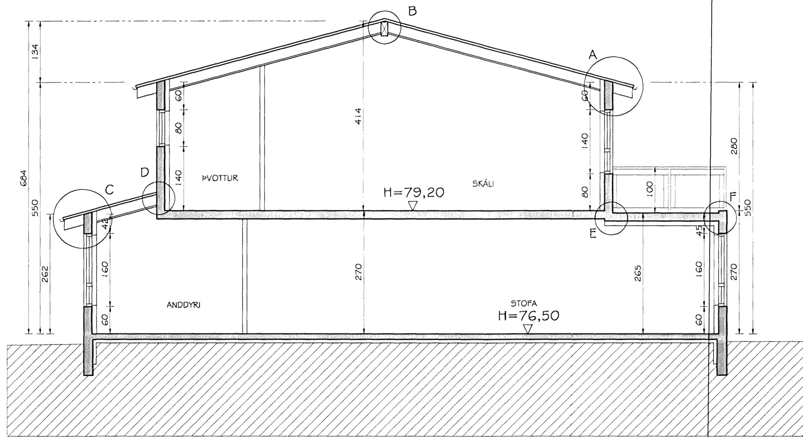
SVÖLUÁS 3 SNIÐ B-B MKV. 1:50
