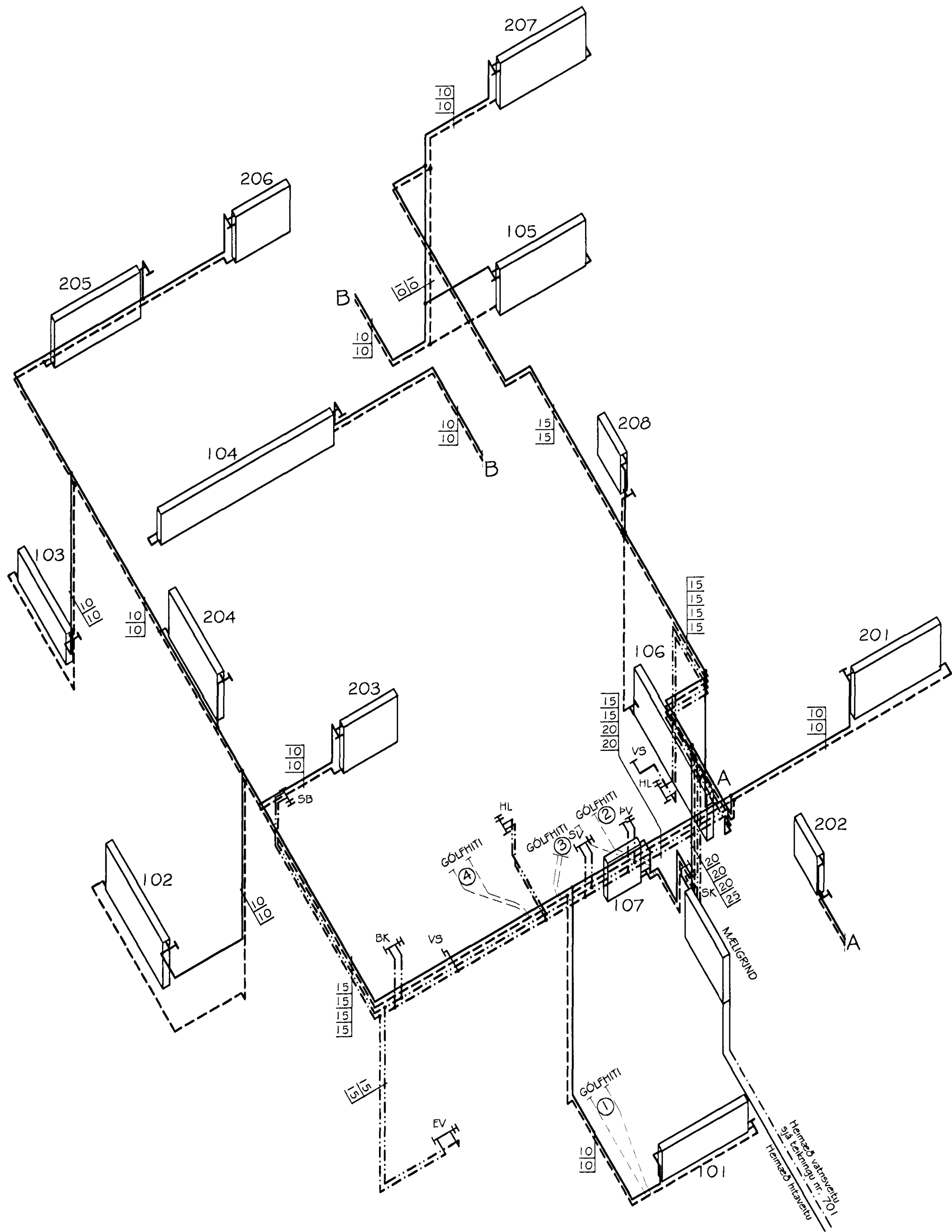
SVÖLUÁS 3 NEYSLUVATNS- OG HITLAGNIR RÚMMYND MKV. 1:50
