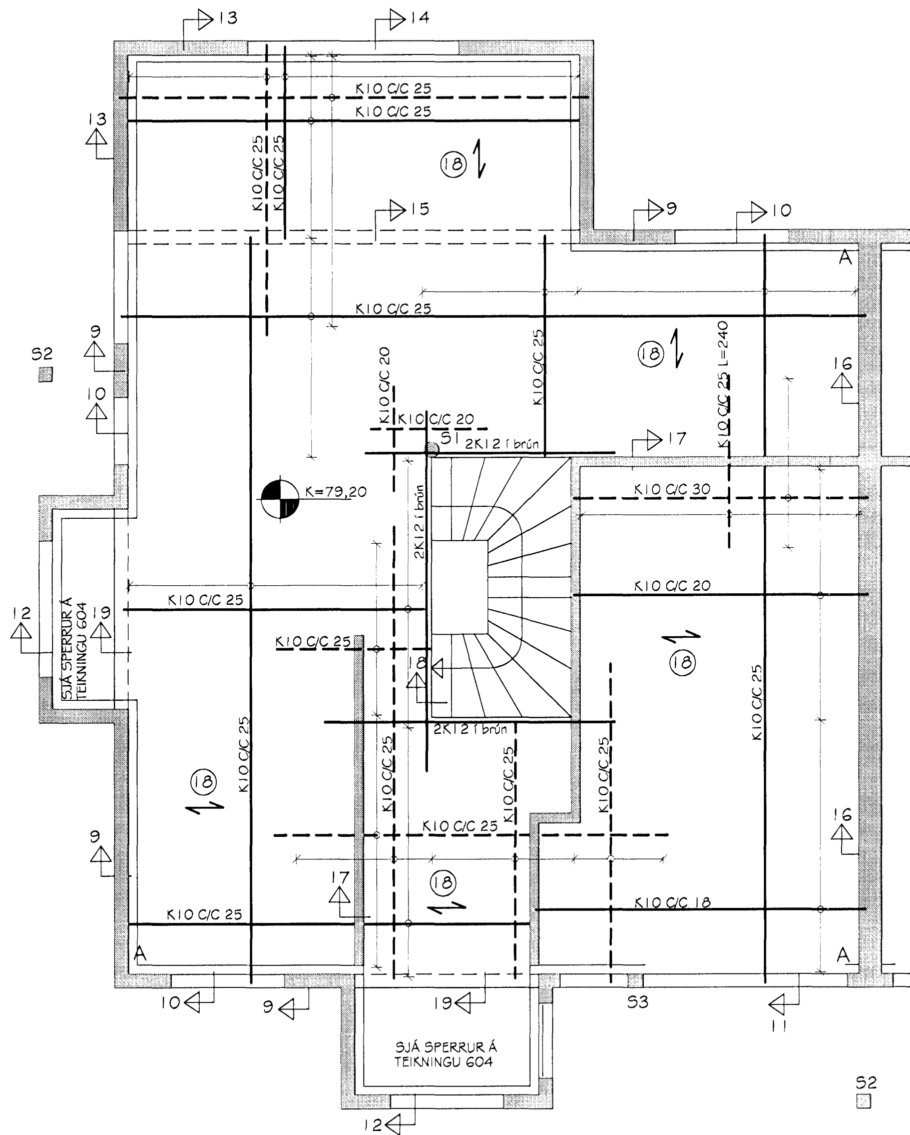
SVÖLUÁS 3 JÁRN Í PLÖTU YFIR 1. HÆÐ GRUNNMYND MKV. 1:50
