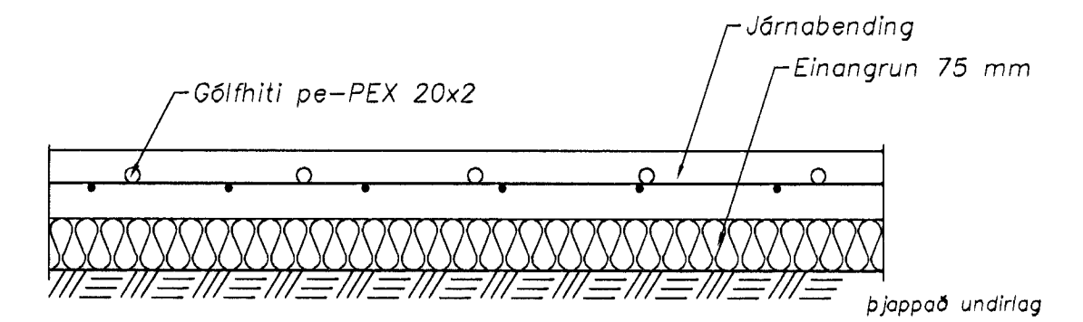
Gólfhiti í botnplötu, Snið 1:10
