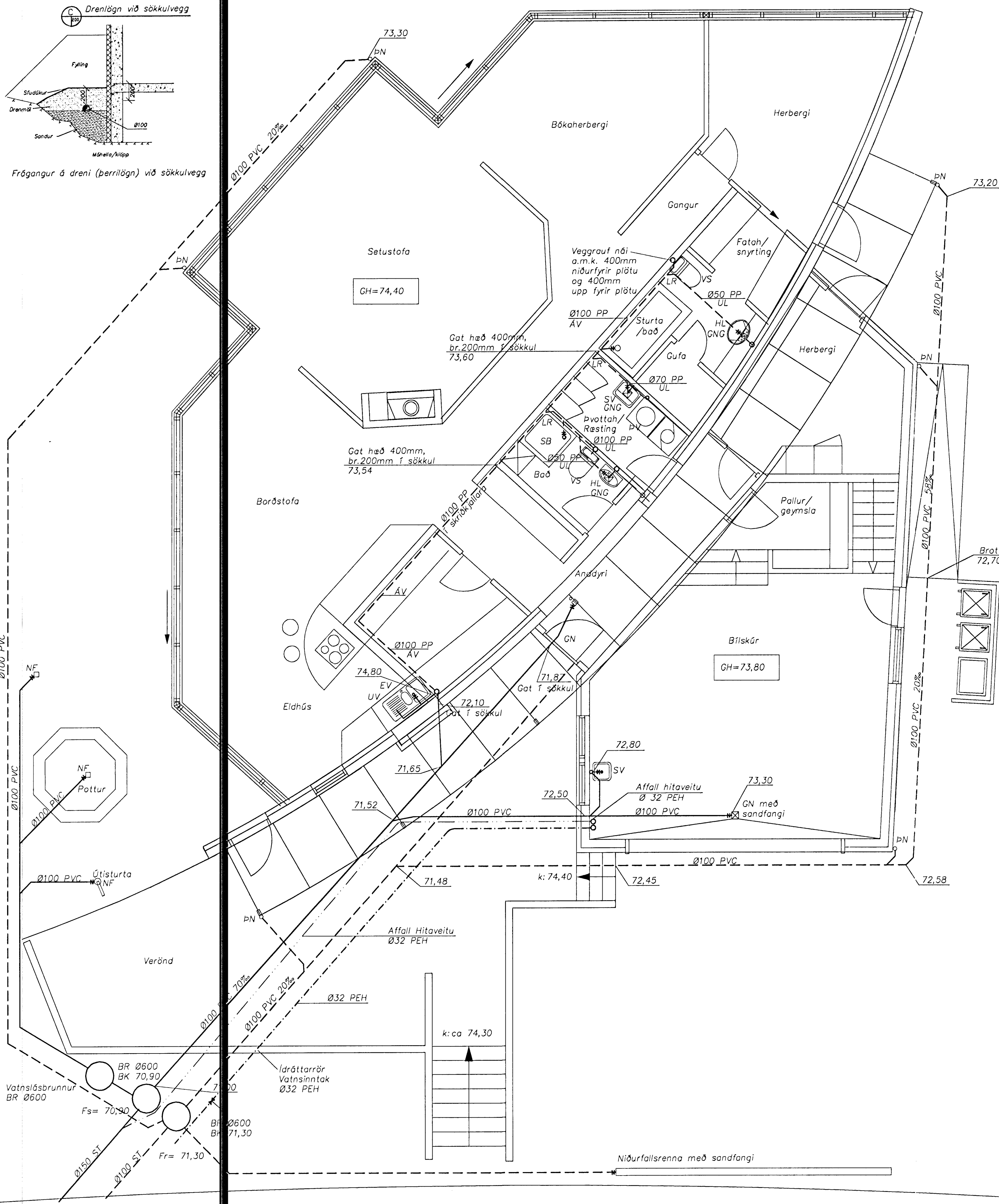
Grunnmynd 1. hæð Málkvarði 1:50
