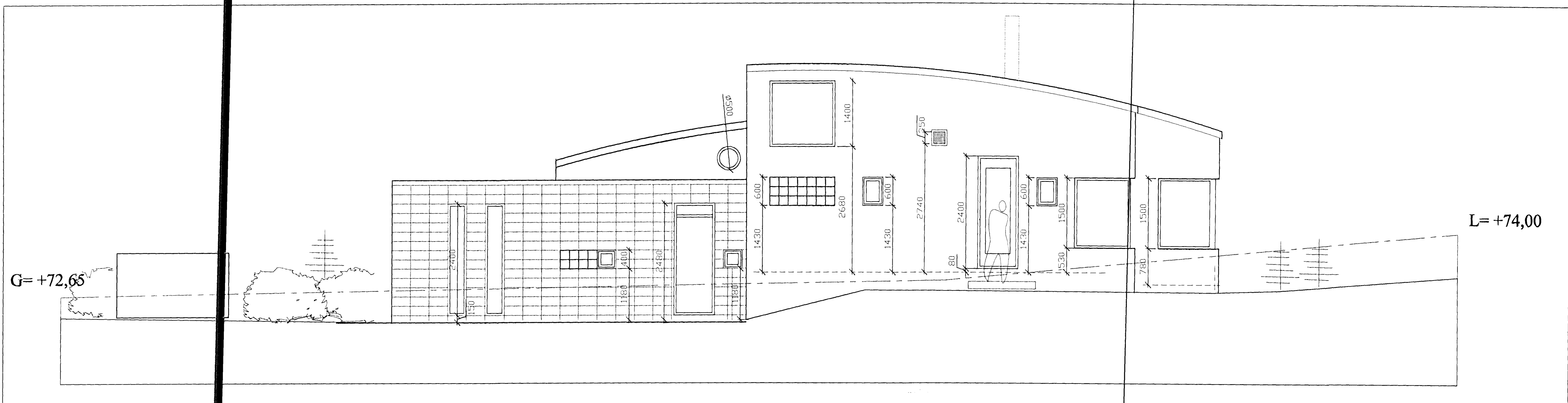
útlit til austur, 1:50
