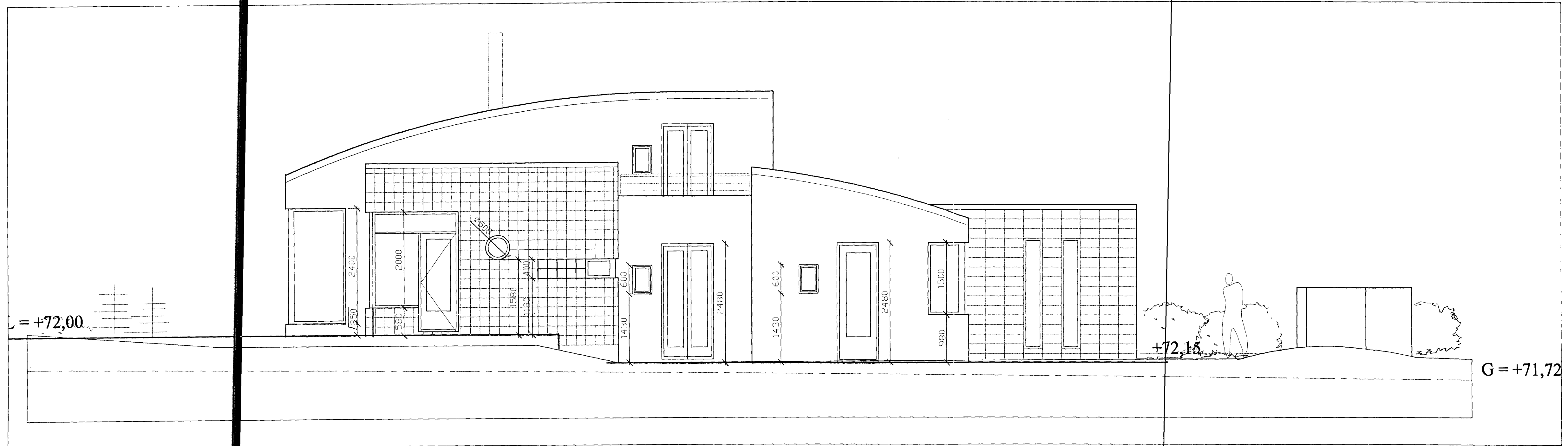
útlit til vesturs, 1:50
