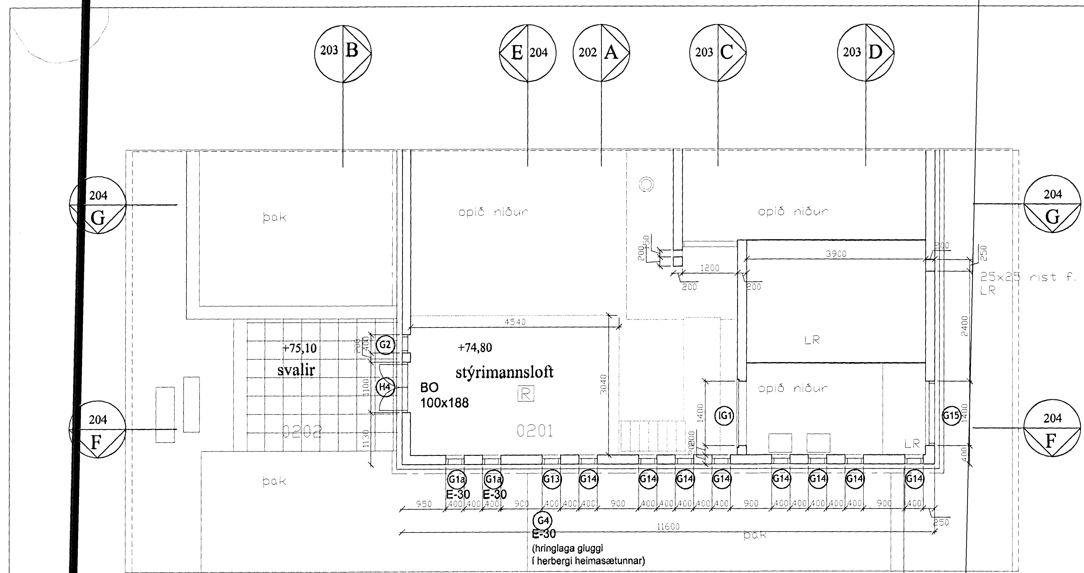
grunnmynd, stýrimannsloft yfir holi 1:50
