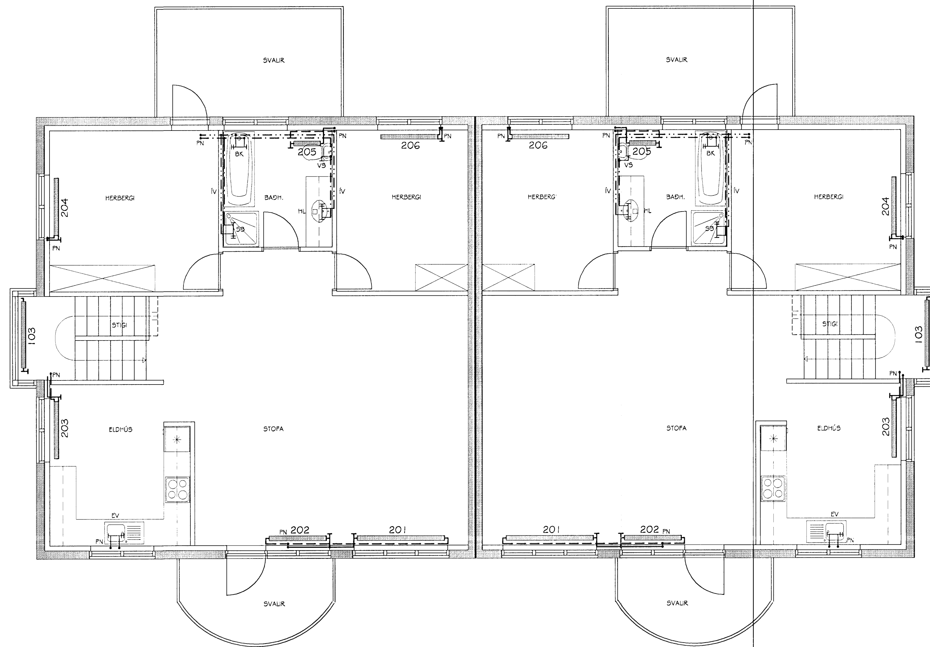
HITA- OG NEYSLUVATNSLAGNIR GRUNNMYND EFRI HÆÐAR MKV. 1:50
