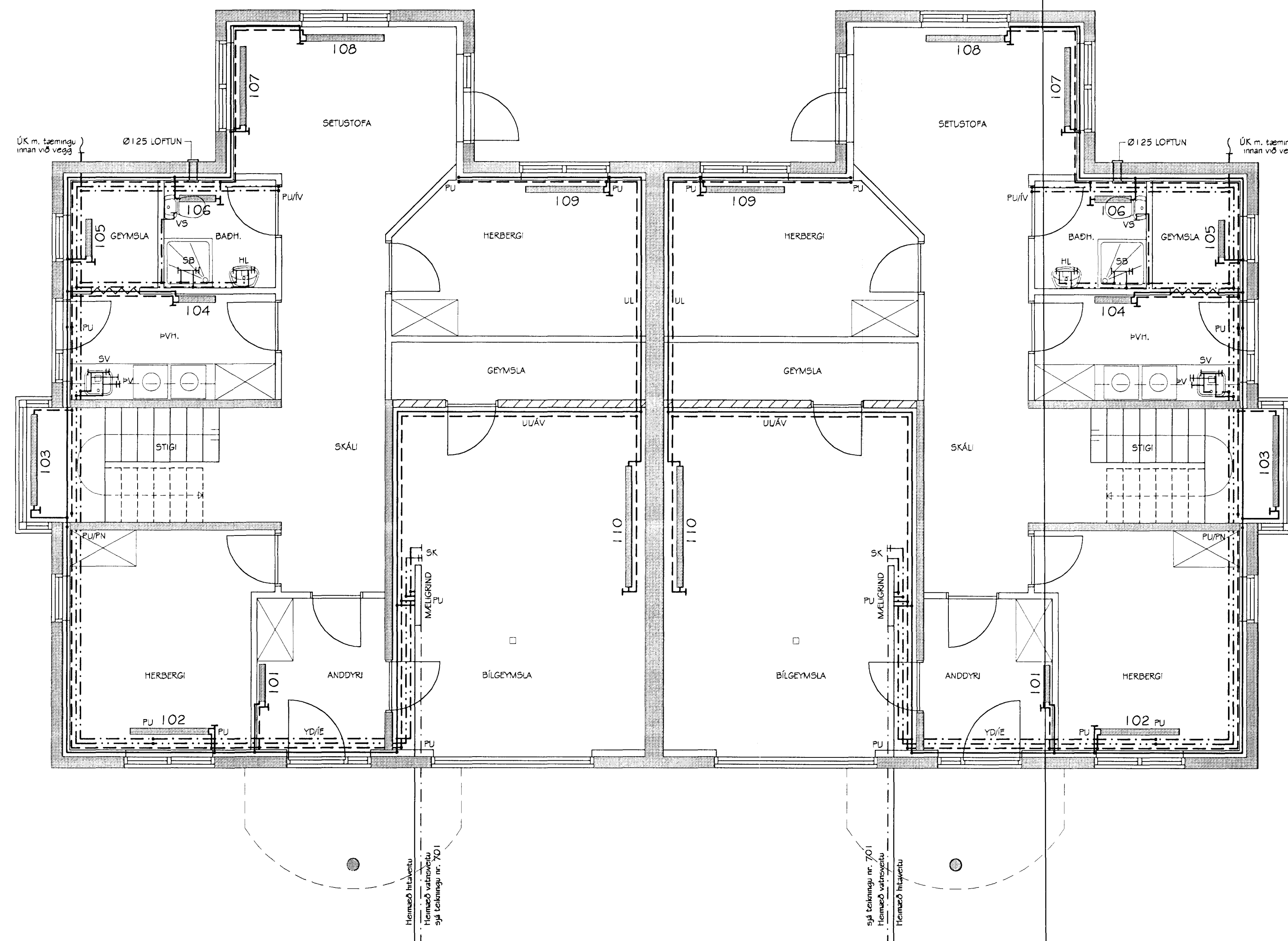
HITA- OG NEYSLUVATNSLAGNIR GRUNNMYND NEDRI HÆÐAR MKV. 1:50
