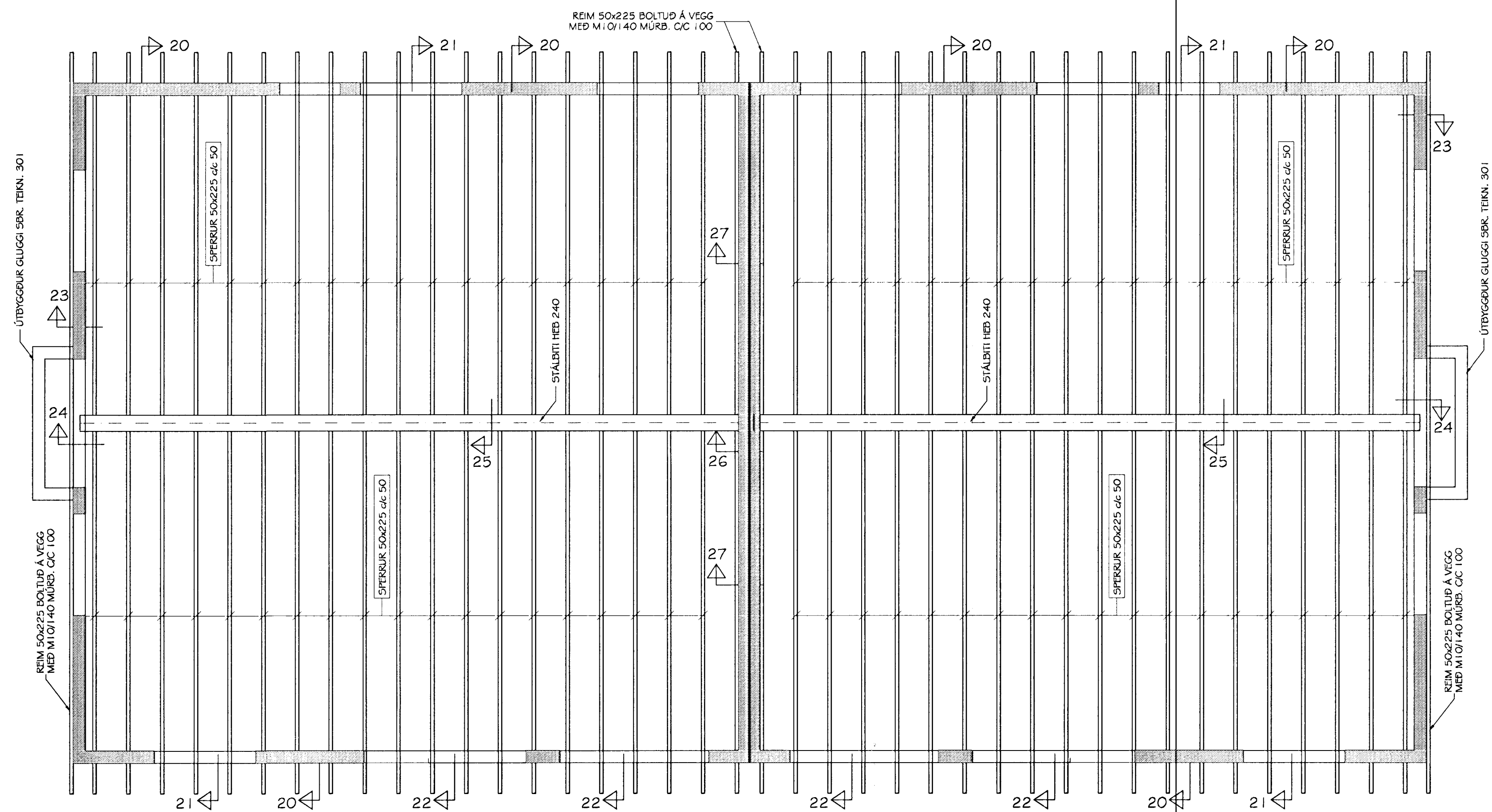
GRUNNMYND ÞAKVIÐA MKV. 1:50
