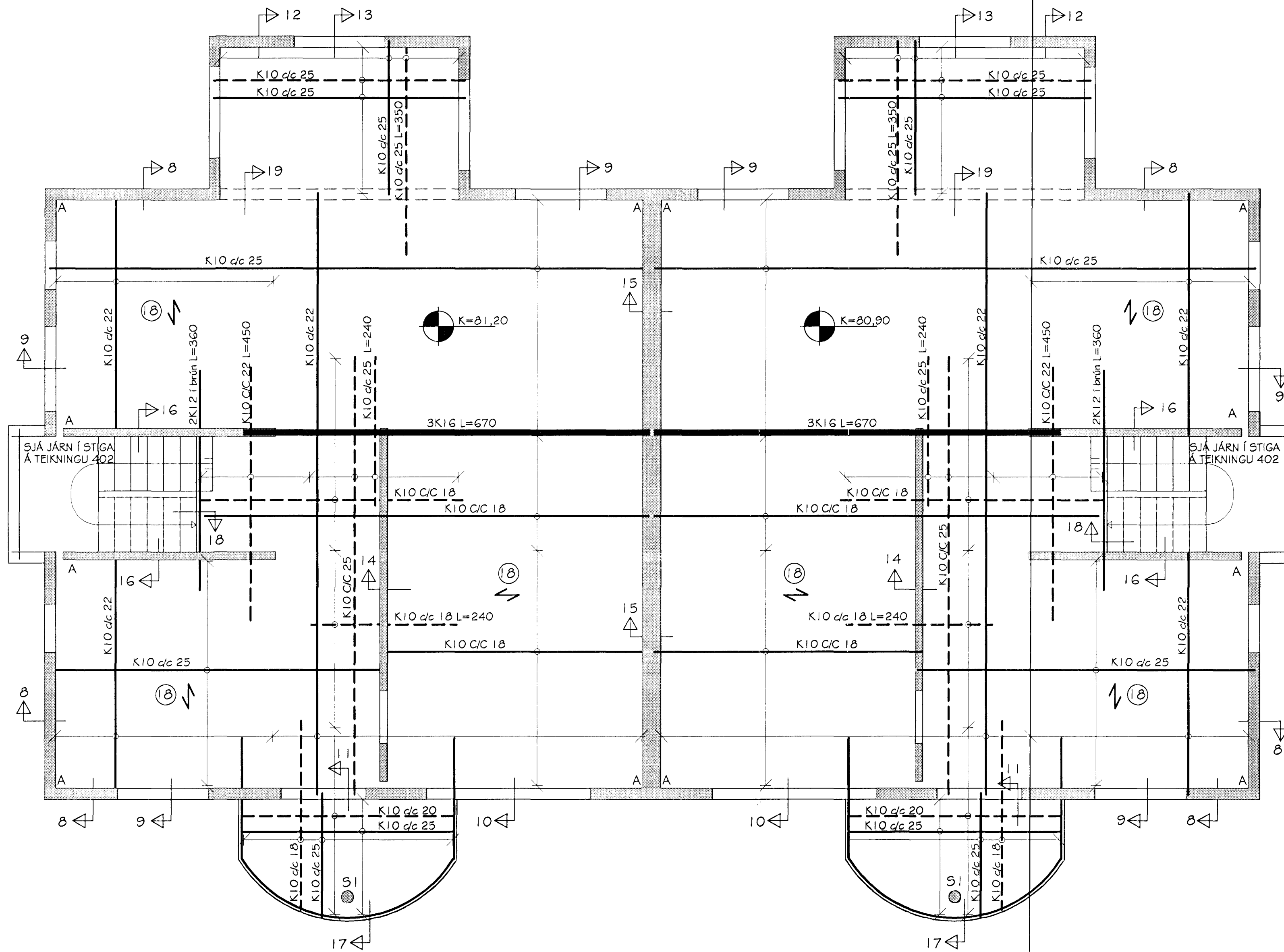
JÄRN Í PLÖTU YFIR NEDRI HÆÐ GRUNNMYND MKV. 1:50
