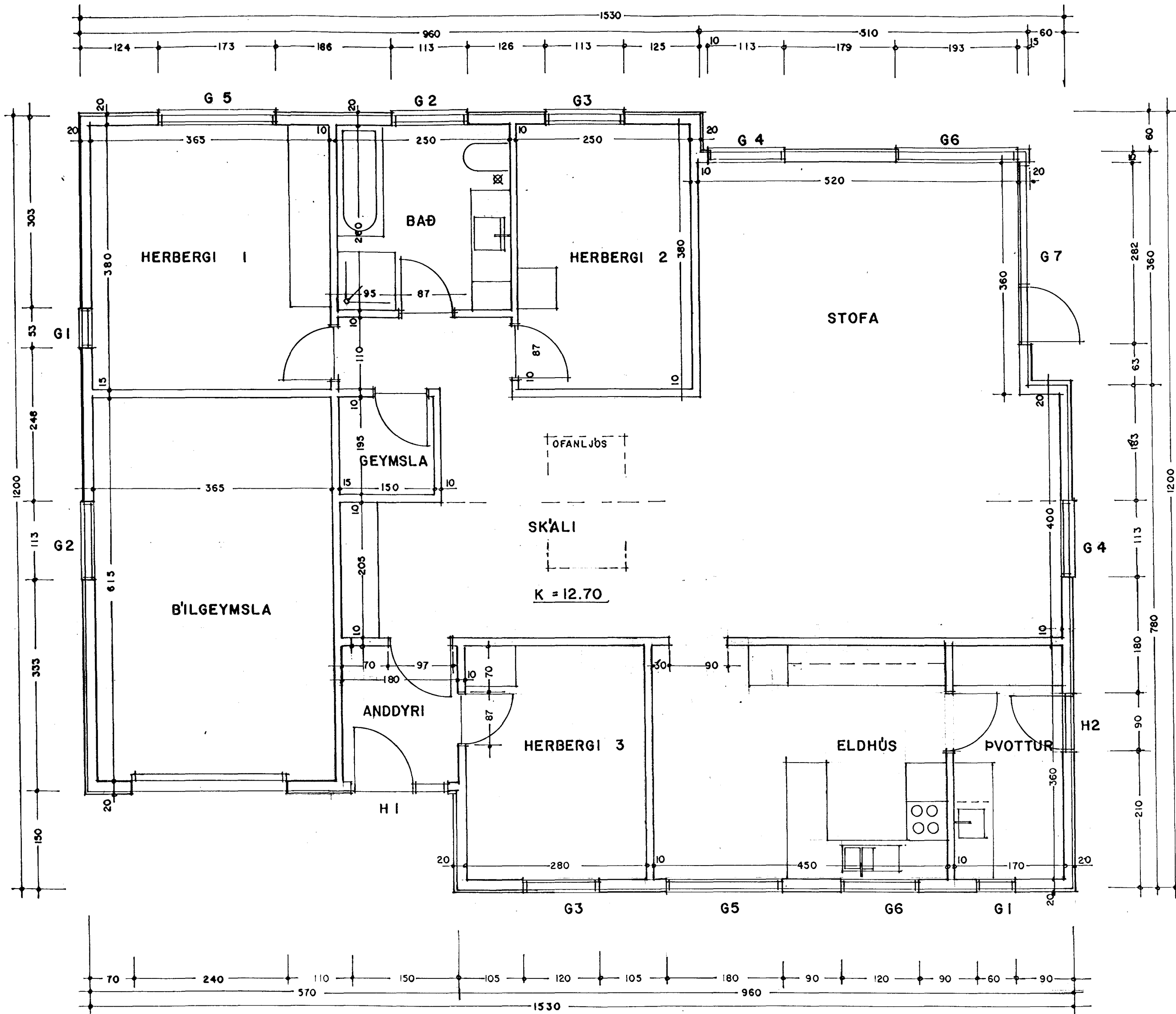
GRUNNMYND 1:50
