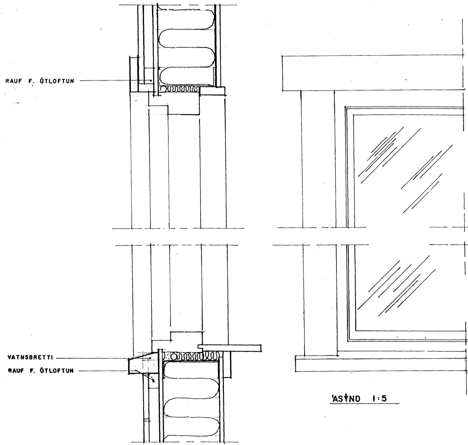
SNEIÐING UM GLUGGA 1:5
