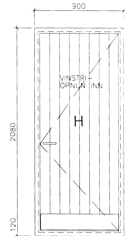
1 STK. HURD OPN. INN (VINSTRI)
