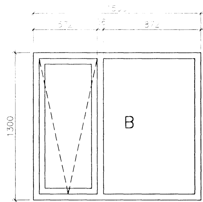
4 STK. GLUGGAR-OPNANLEGIR
