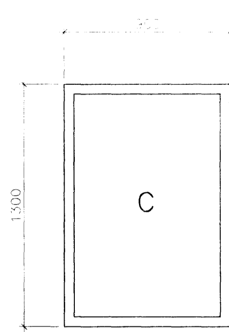
3 STK. GLUGGAR
