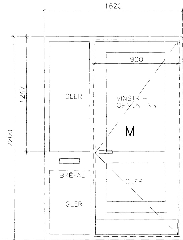
1 STK. HURD OPN. INN (VINSTRI)
