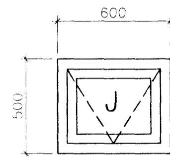
1 STK. GLUGGI-OPNANLEGUR
