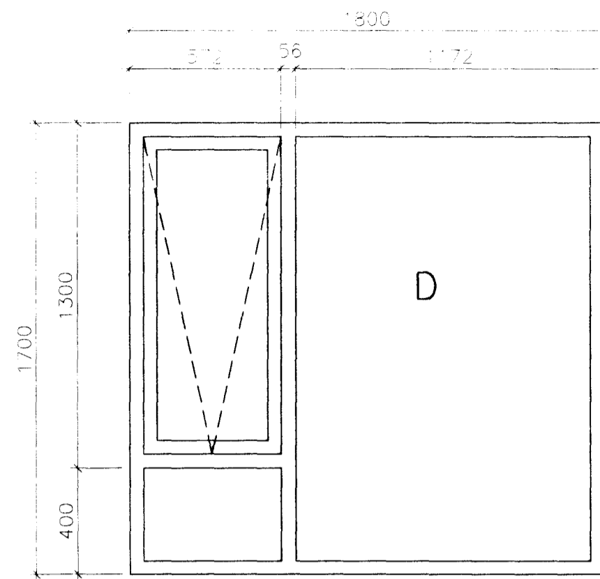
1 STK. GLUGGI-OPNANLEGUR
