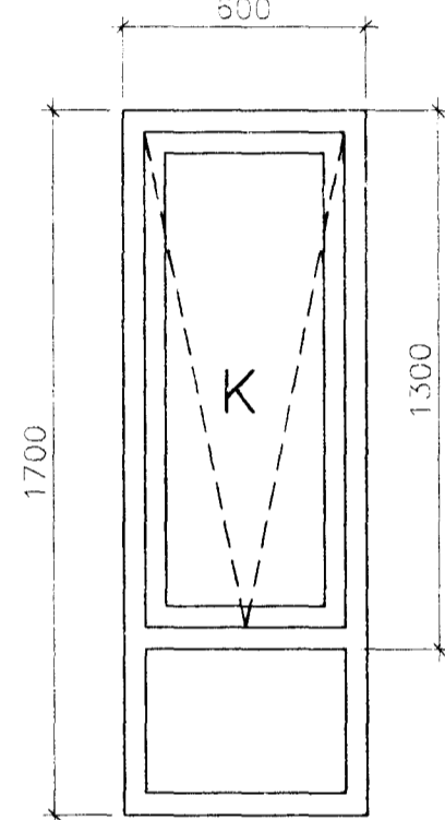
1 STK. GLUGGI-OPNANLEGUR
