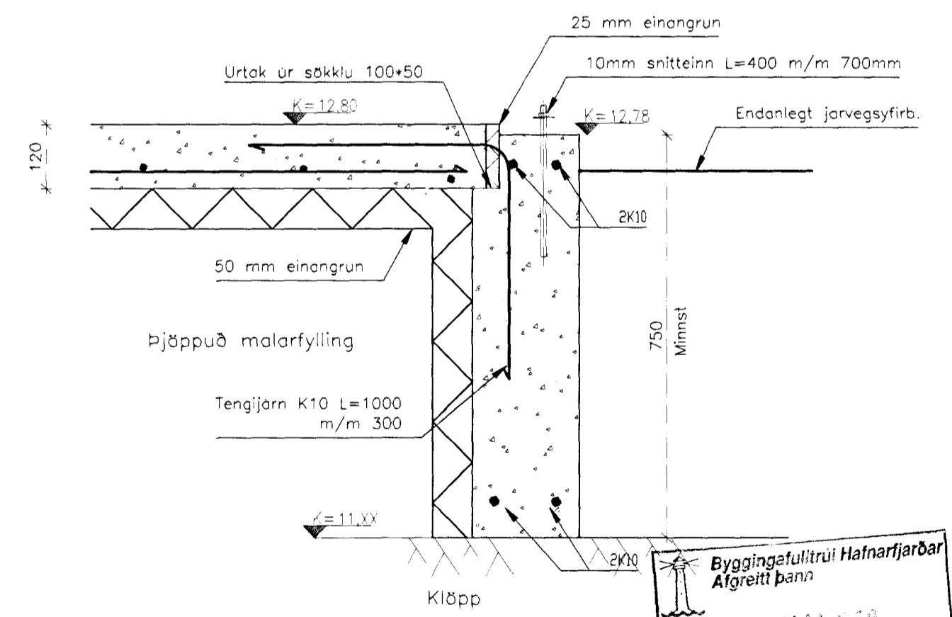
01 SKURÐUR I ÚTVEGG Mkv: 1/10
