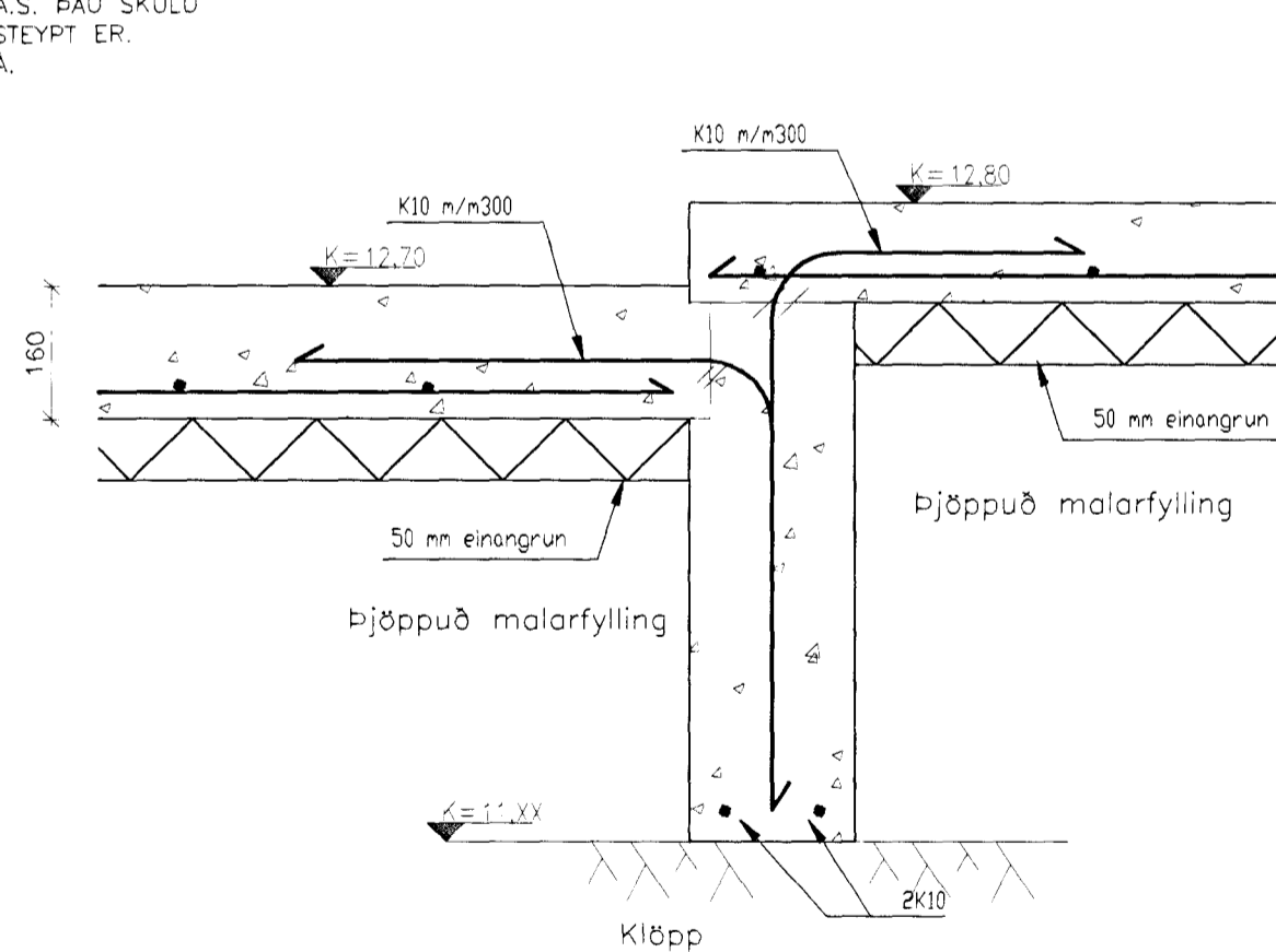
03 SKURÐUR I MILLIVEGG BILGEYMSLU Mkv: 1/10
