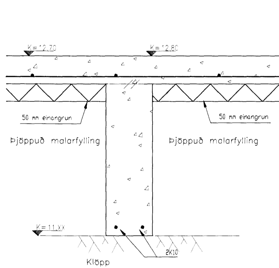
02 SKURÐUR I INNVEGG Mkv: 1/10
