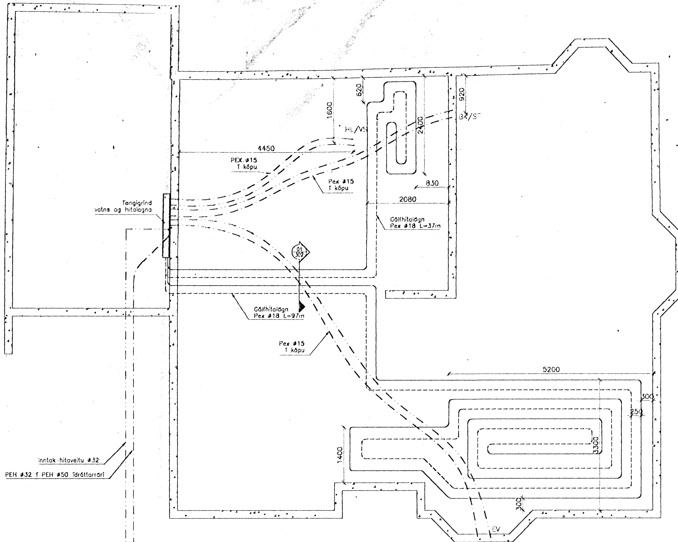
GRUNNMYND HITA OG NEYSLUVATNSLAGNA Í PÖTU Mkv: 1/50
