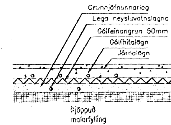
STADSETNING HITA OG NEYSLUVATNSLAGNA Í PÖTU Mkv: 1/20
