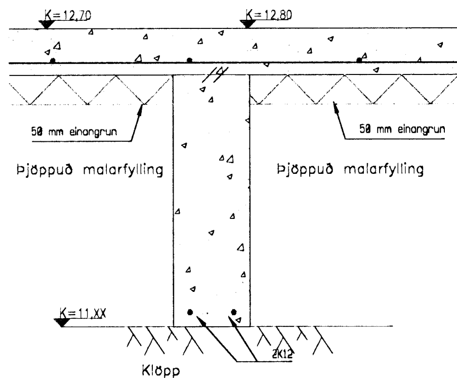
02 SKURÐUR Í INNVEGG Mkv: 1/10
