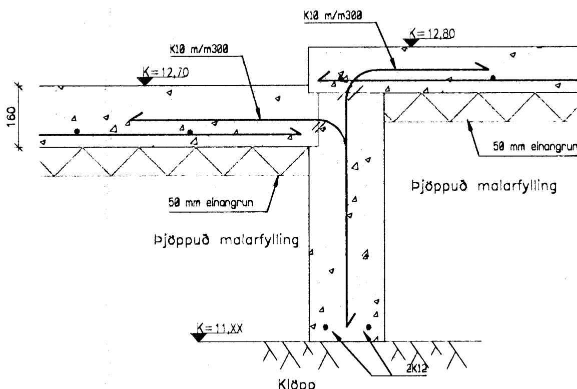
03 SKURÐUR Í MILLIVEGG BILGEYMSLU Mkv: 1/10
