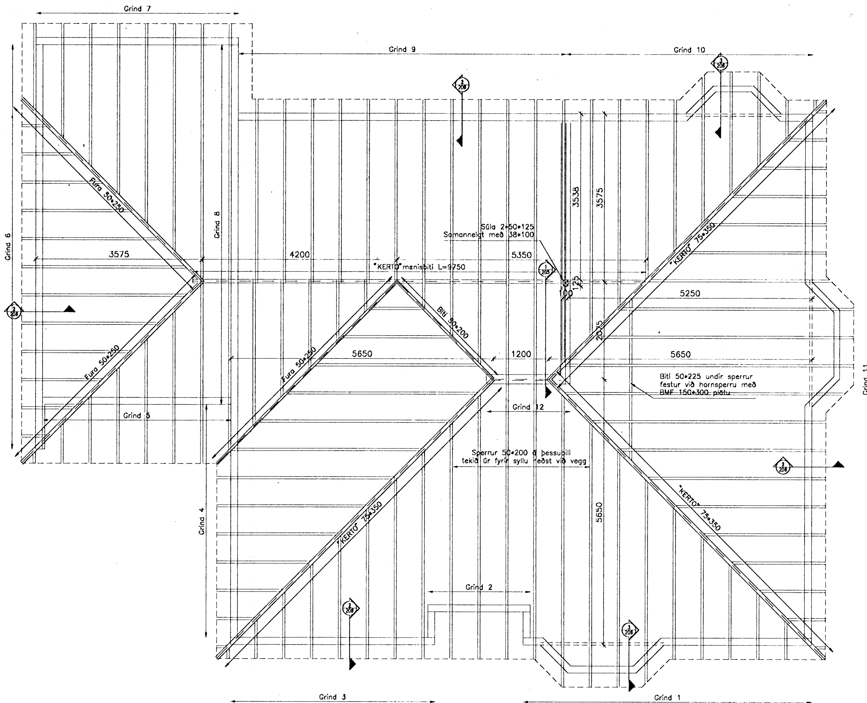
GRUNNMYND SPERRA OG VEGGRINDA Mkv: 1/50
