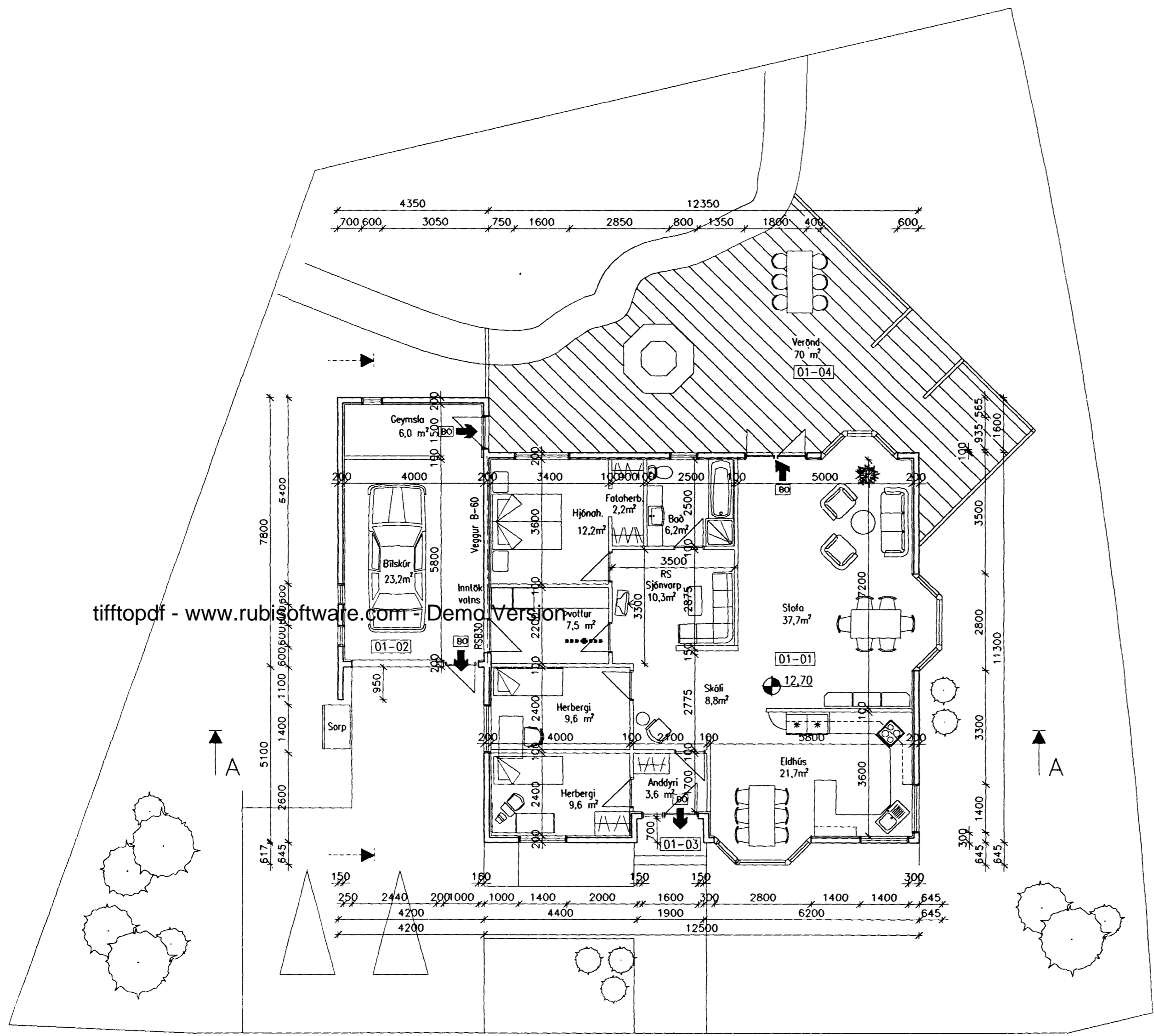
GRUNNMYND Mkv: 1/100
