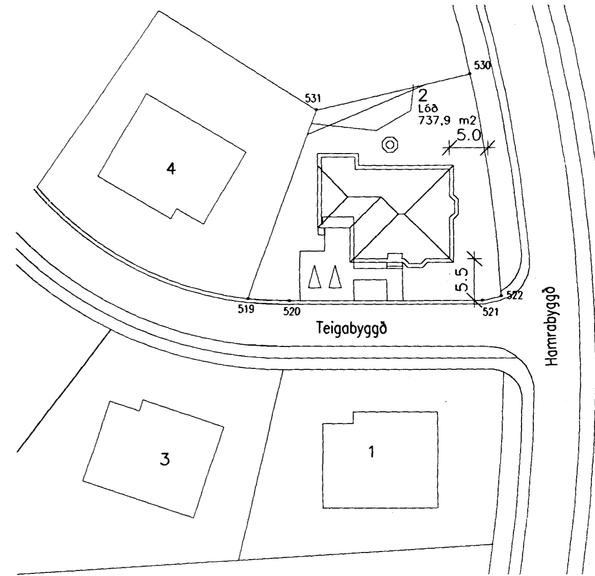
AFSTÖÐUMYND Mkv: 1/500
