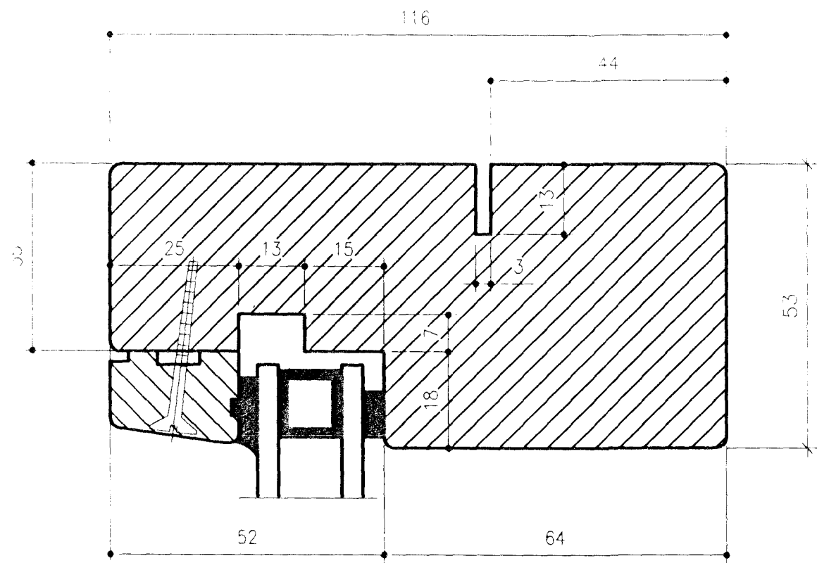
HLIDAR/YFIRSTYKKI (GLUGGA)
