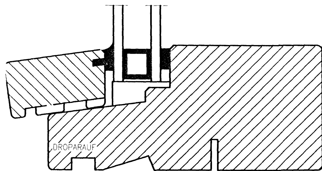
UNDIRSTYKKI (GLUGGA)
