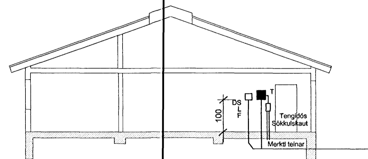
Snið a-a mkv. 1:100
