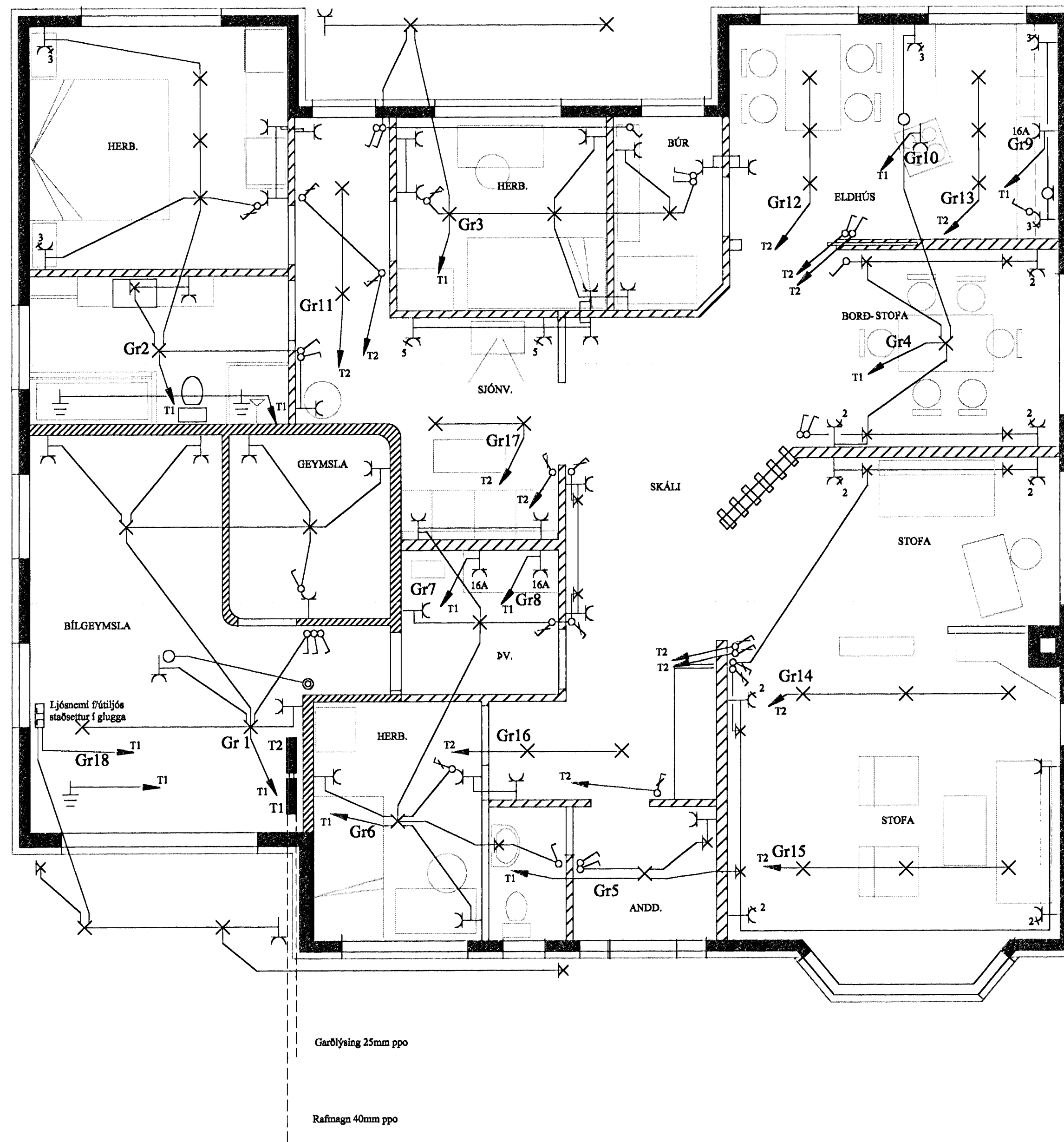
Grunnmynd 1:50
