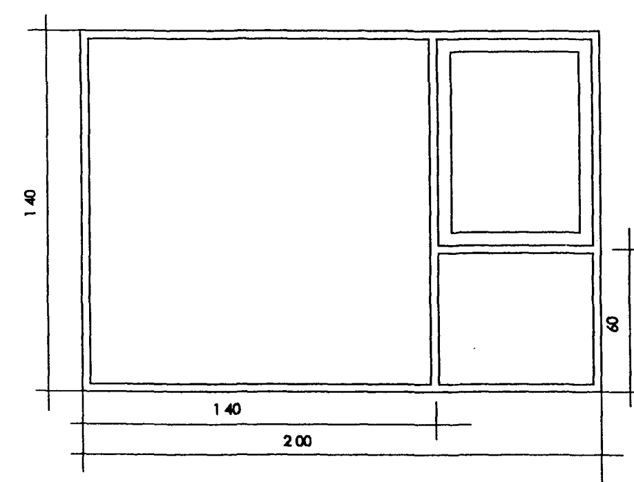
GLUGGI # 7. 1 STK.
