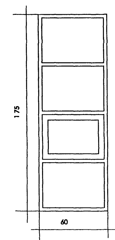
GLUGGI # 2. 1 STK.
