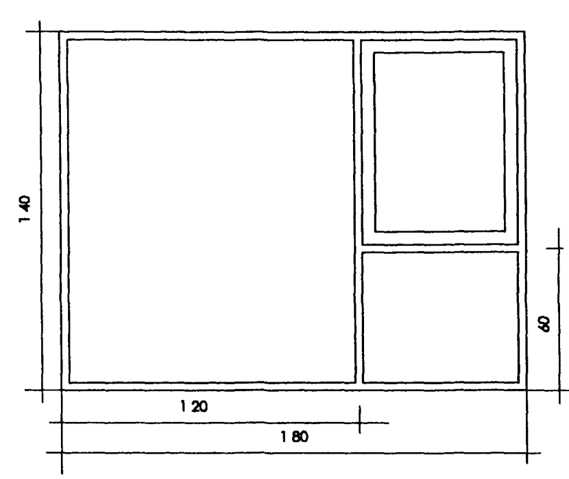
GLUGGI # 6. 2 STK.
