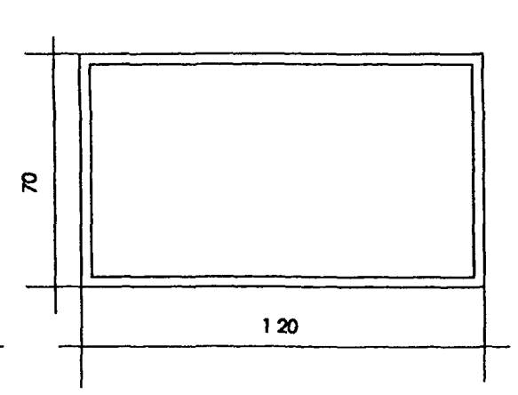
GLUGGI # 10. 1 STK.
