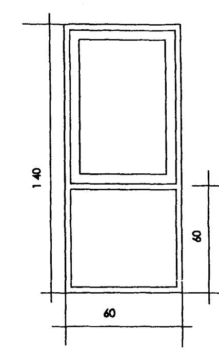
GLUGGI # 8. 1 STK.
