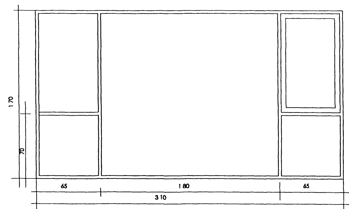
GLUGGI # 1. 1 STK.
