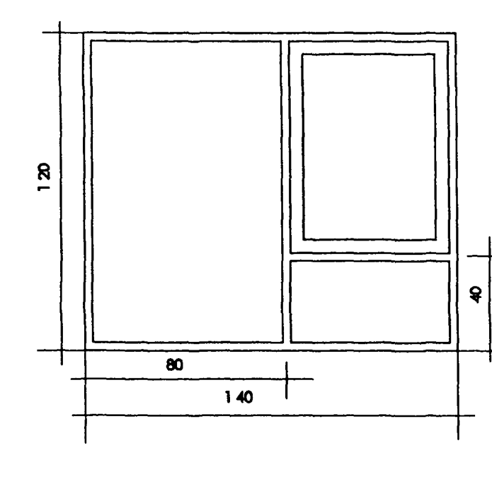
GLUGGI # 5. 2 STK.
