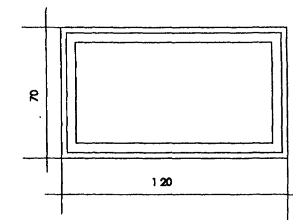
GLUGGI # 9. 2 STK.
