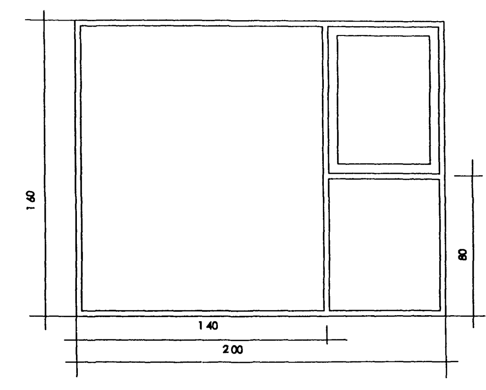
GLUGGI # 4. 1 STK.
