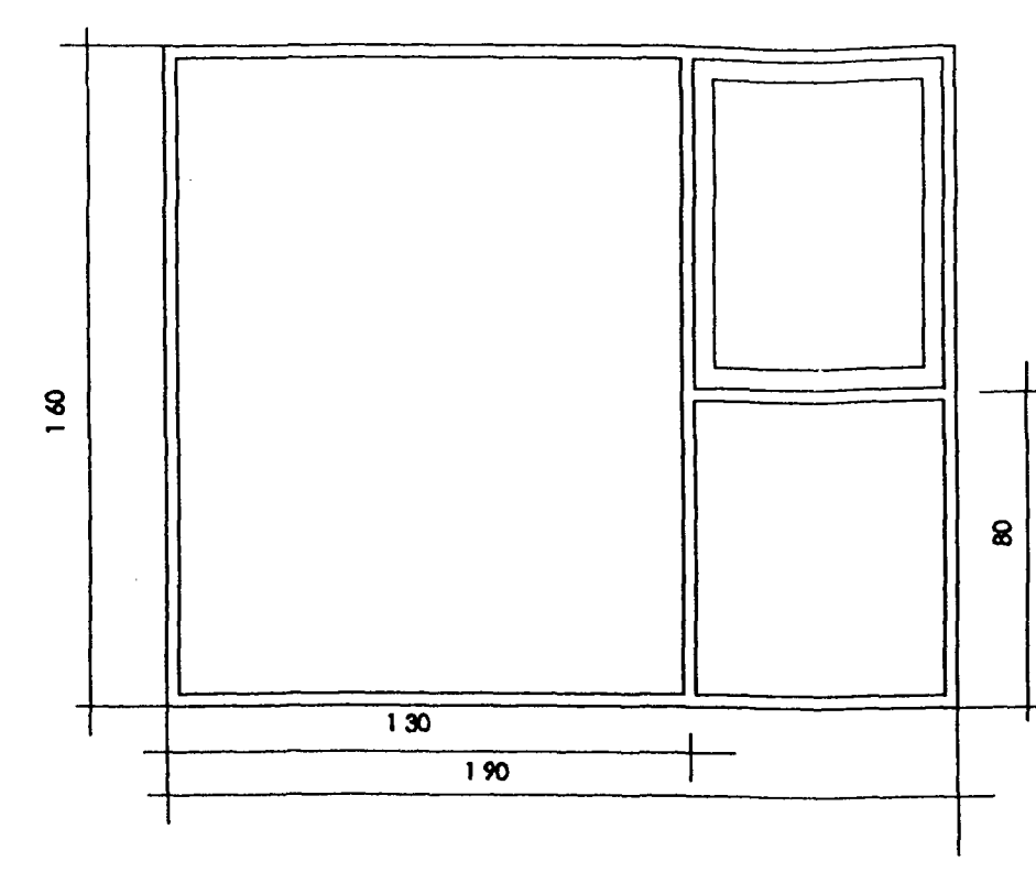
GLUGGI # 3. 1 STK.
