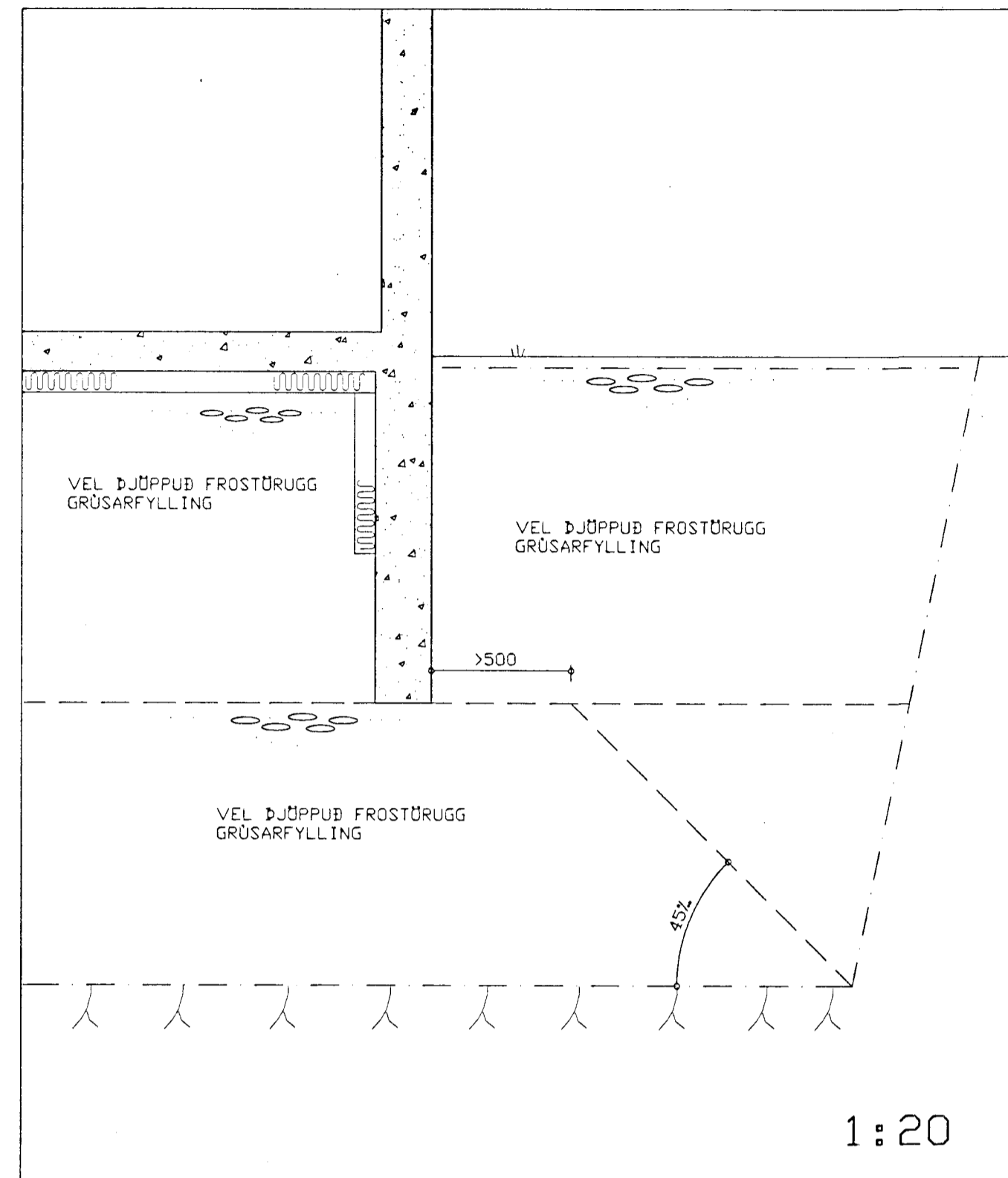
SNIÐ A-A
