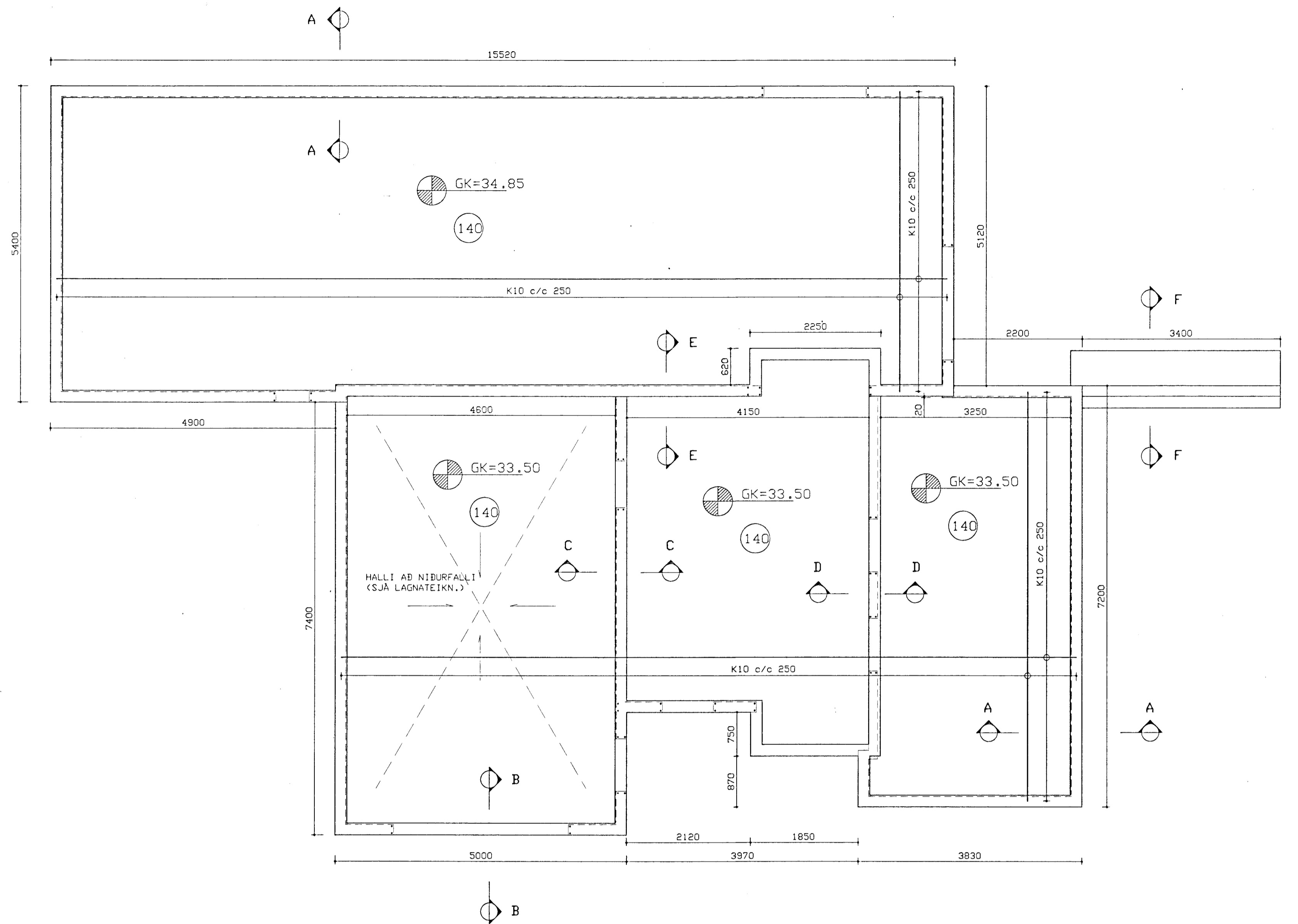
GRUNNMYND 1:100 JARÐHÆÐ OG MILLIHÆÐ
