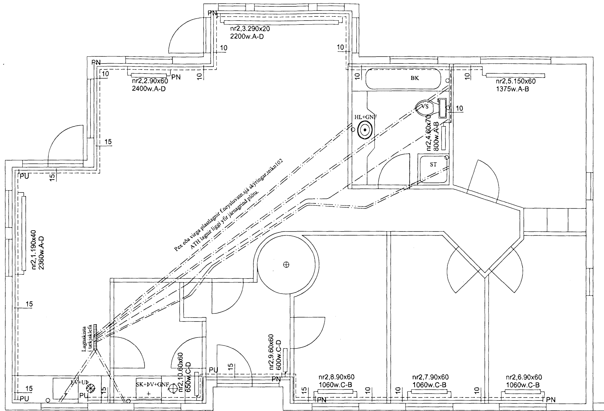
Grunnmynd hita- og neysluvatnslagna 2.hæðar. mkv.:1:50
