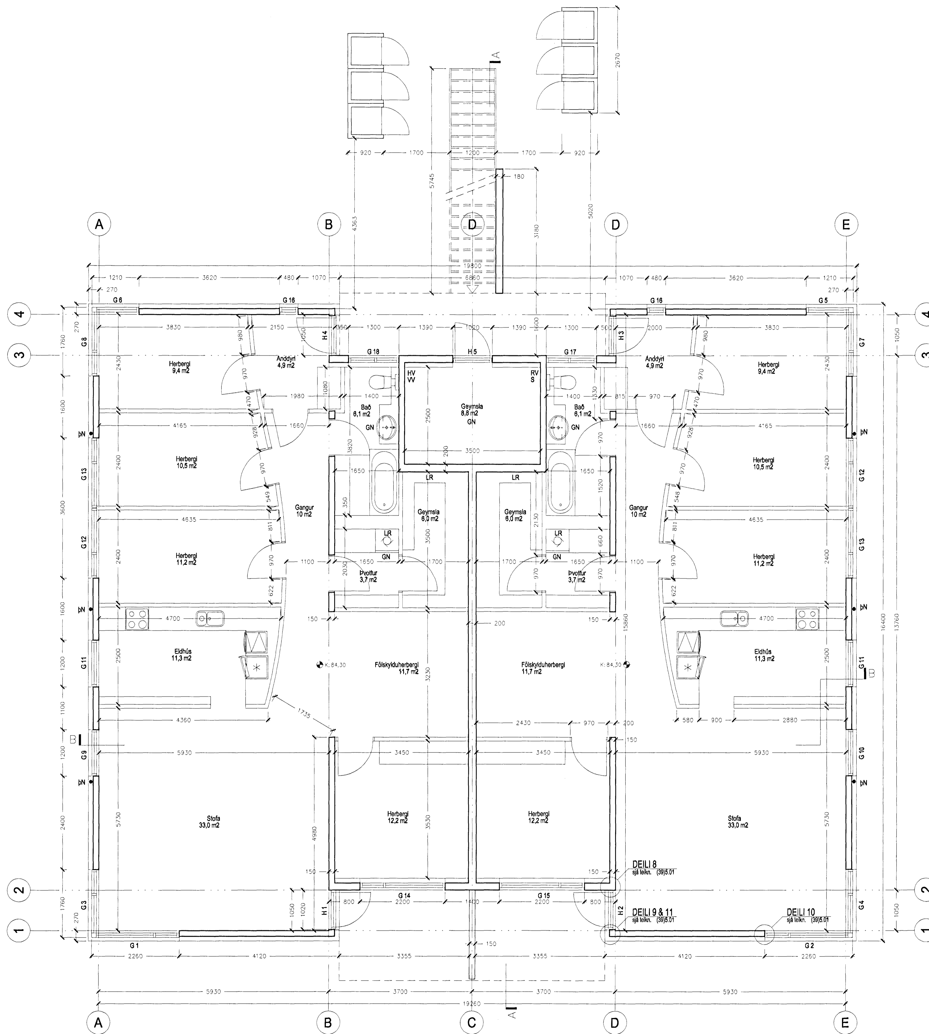
GRUNNMYND 1. HÆÐAR mkv. 1:50
