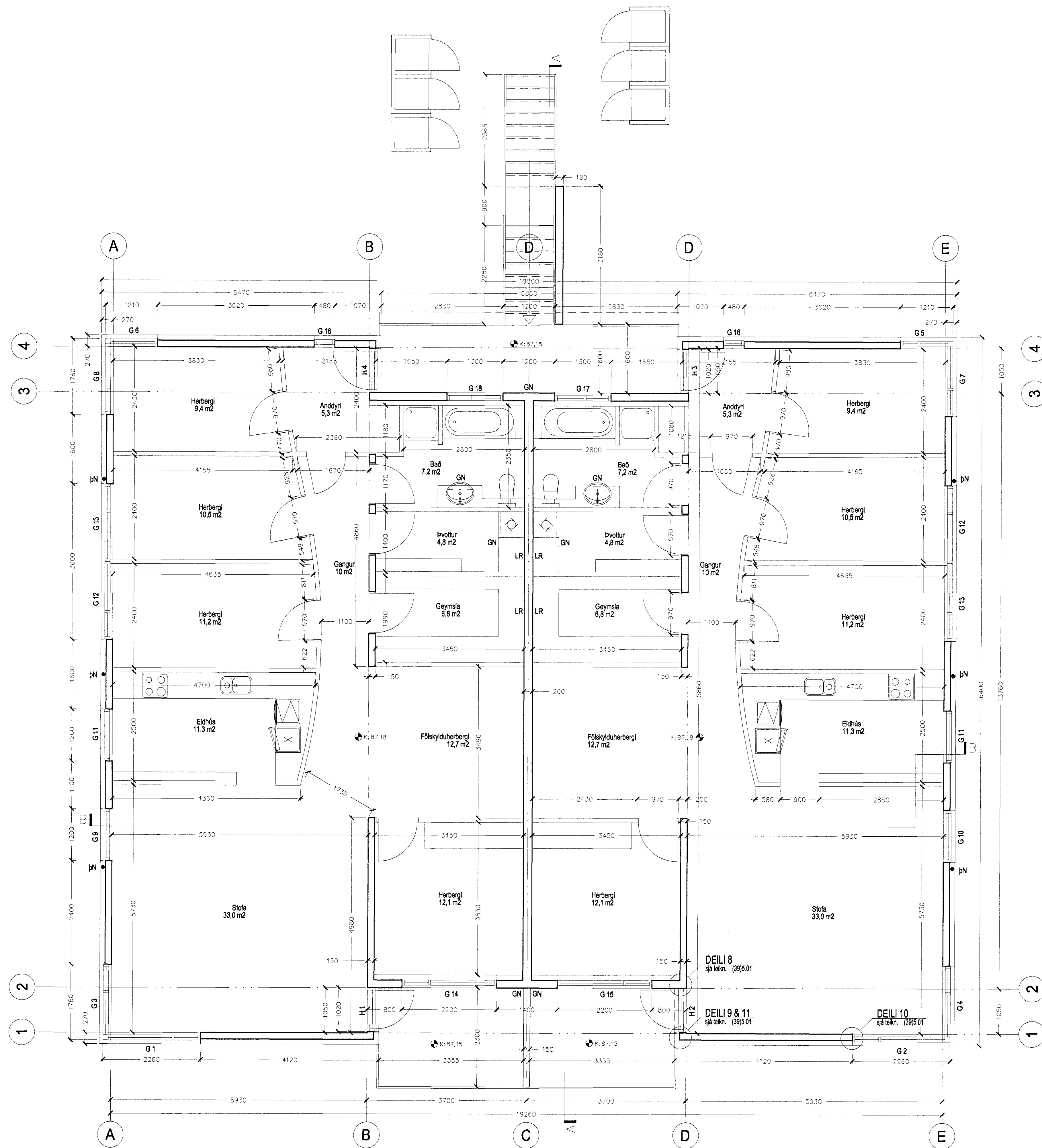
GRUNNMYND 2. HÆÐAR m.kv. 1:50
