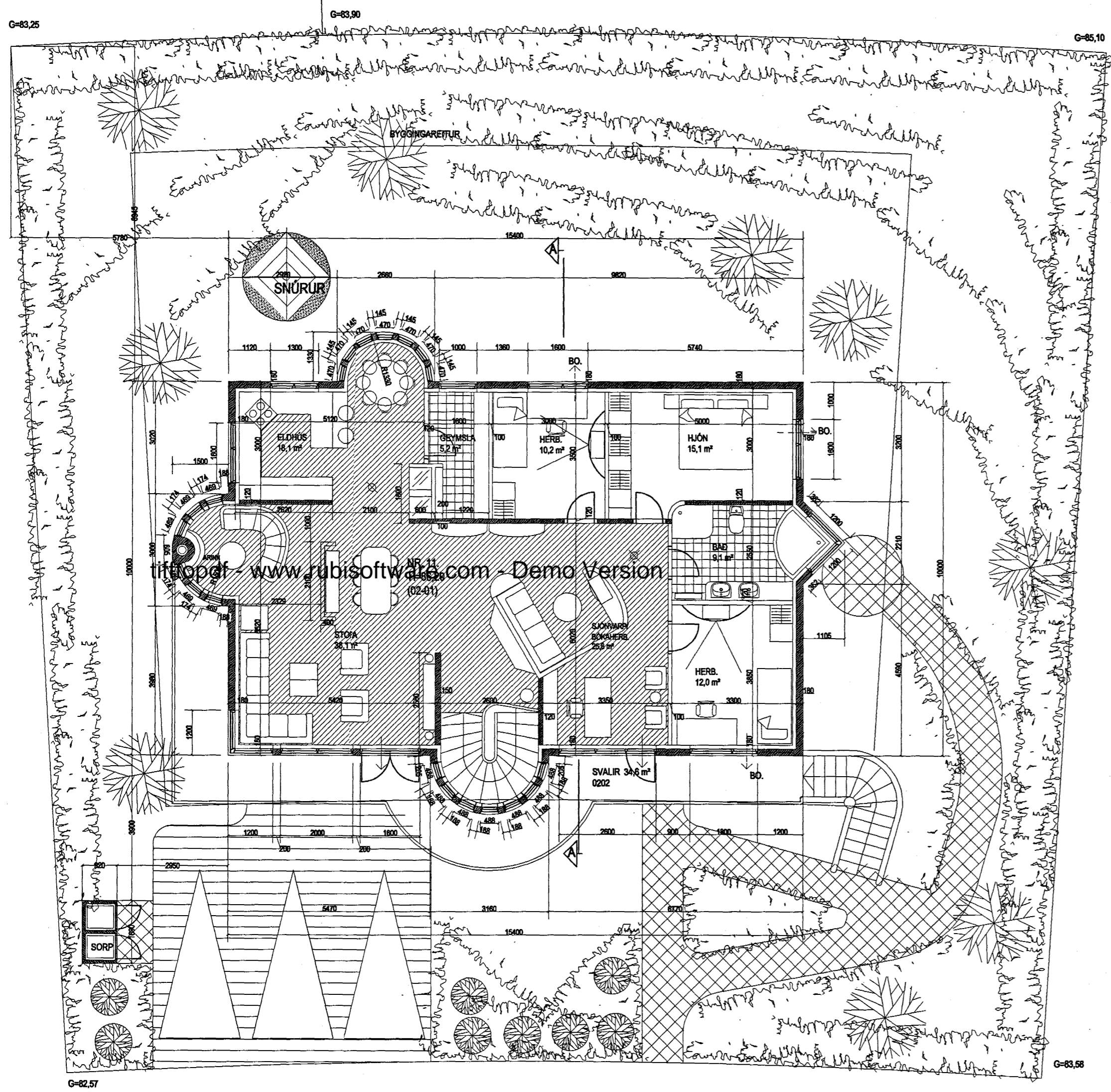
GRUNNMYND 2. HÆÐ MKV 1:100.
