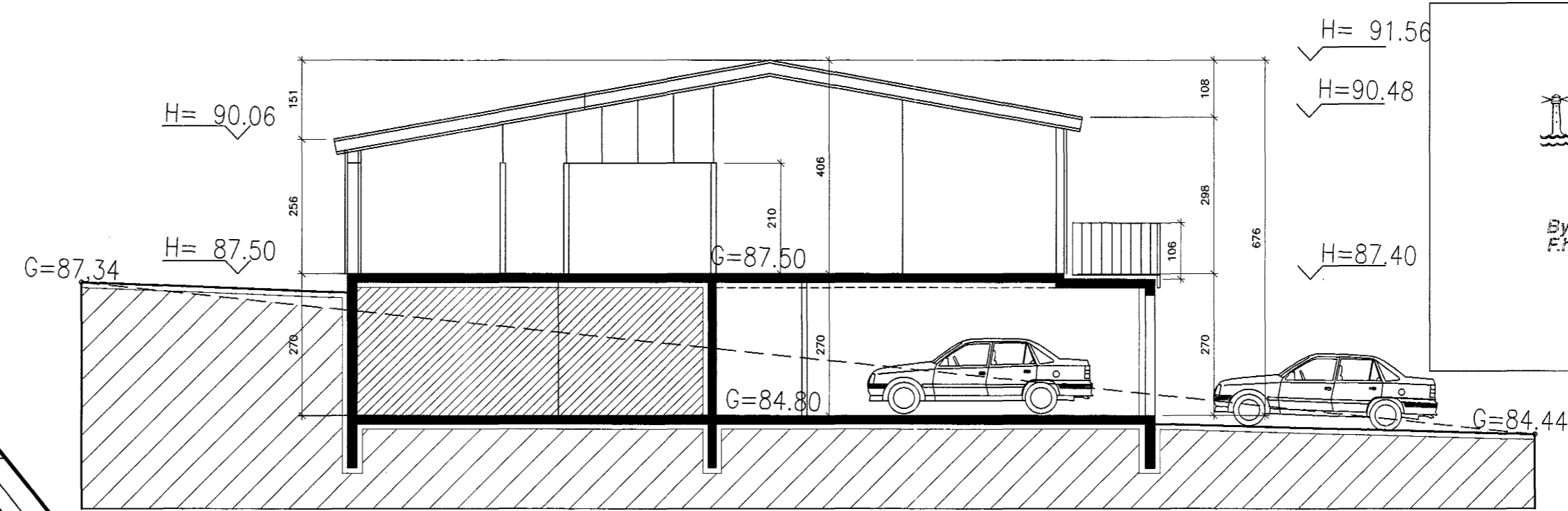
SNEIDING A-A
