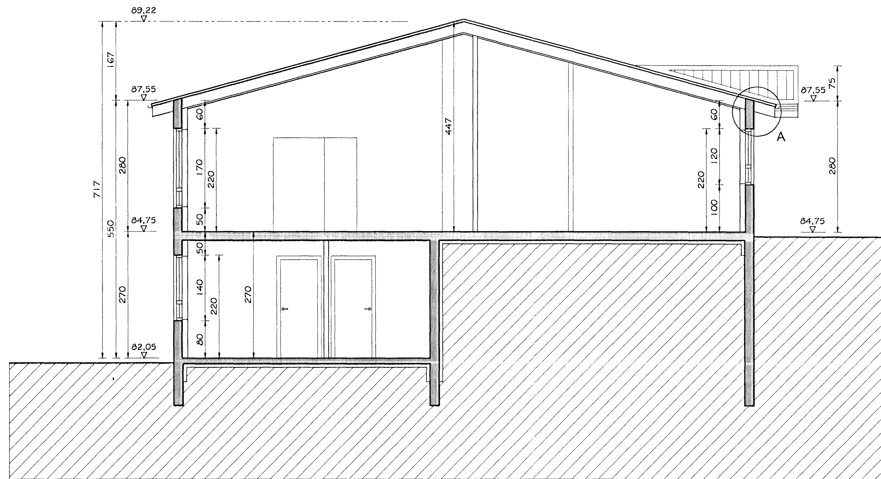
SNID C-C MKV. 1:50
