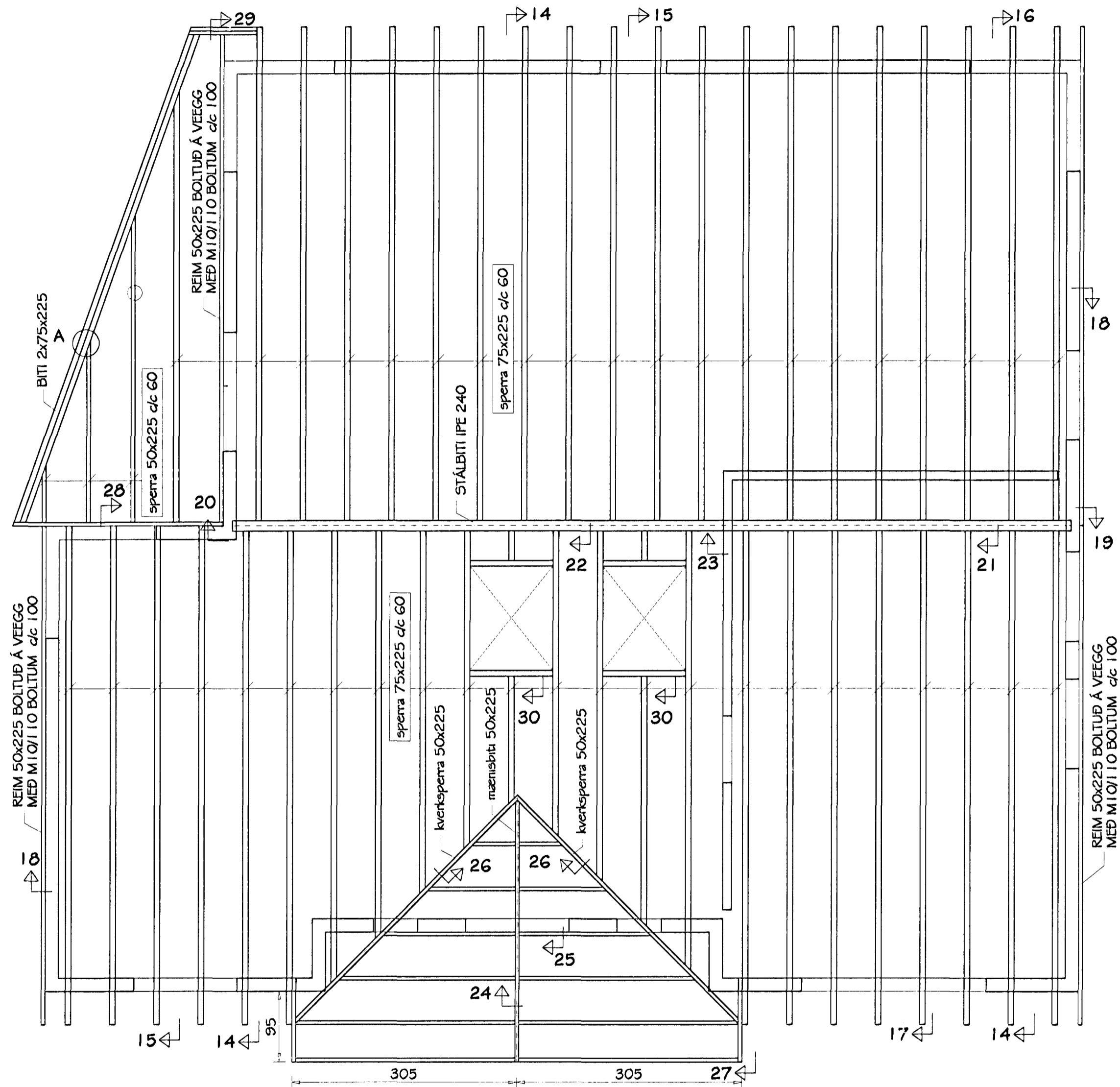
ÞAKVIÐIR - GRUNNMYND MKV. 1:50
