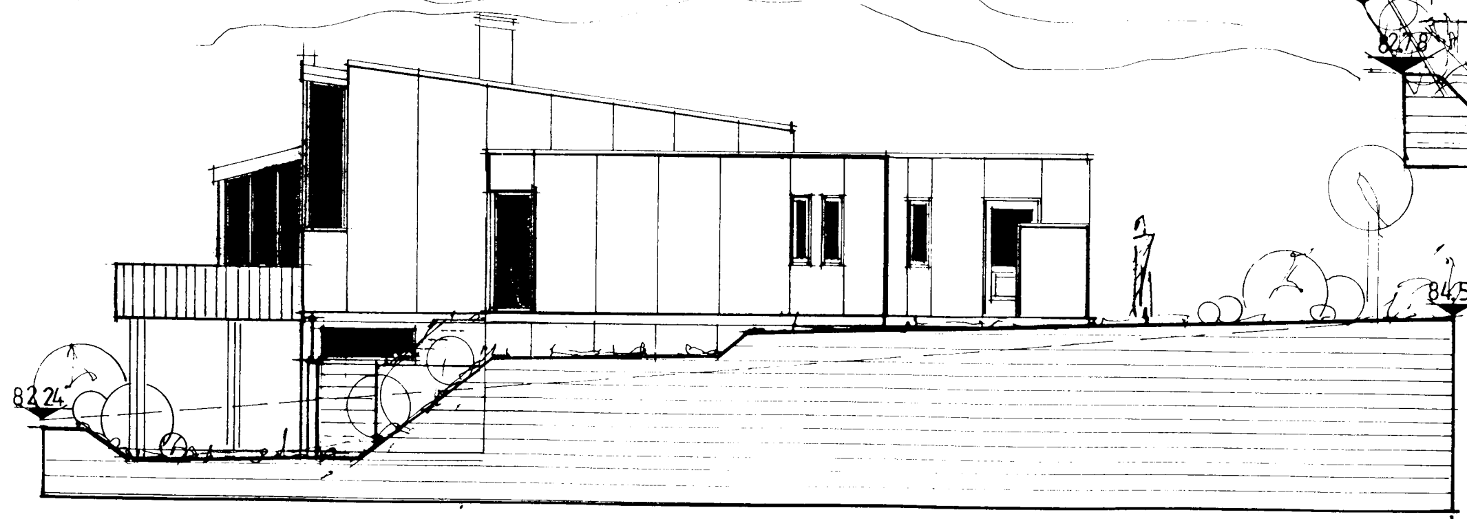
AUSSLÆG HLIÐ 1:100
