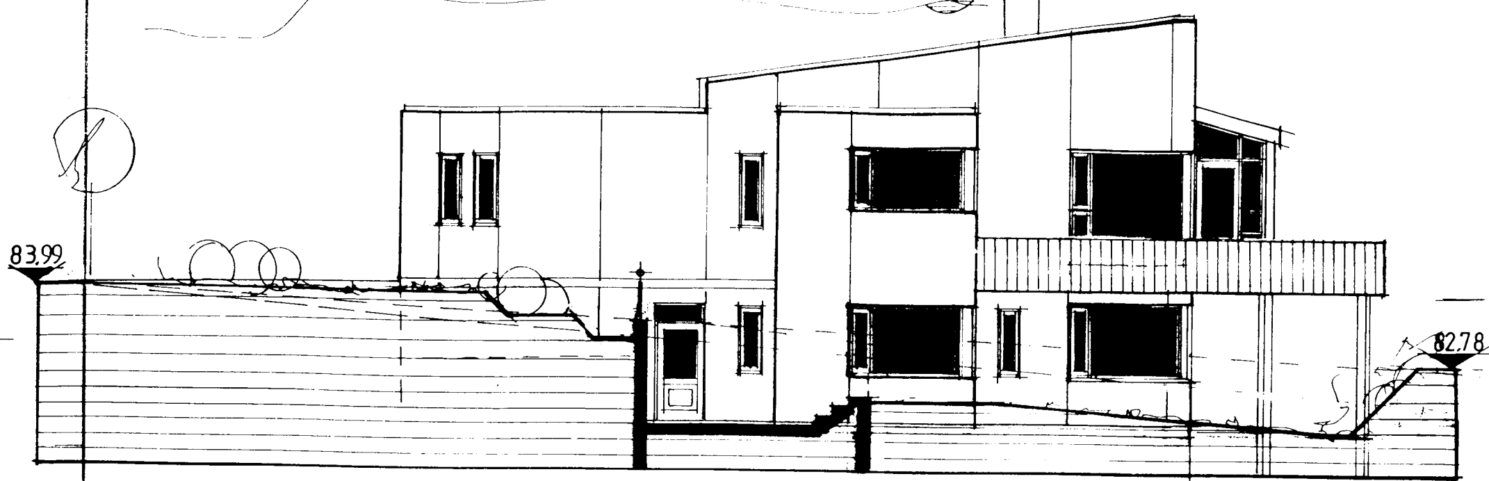
VESTLÆG HLIÐ 1:100
