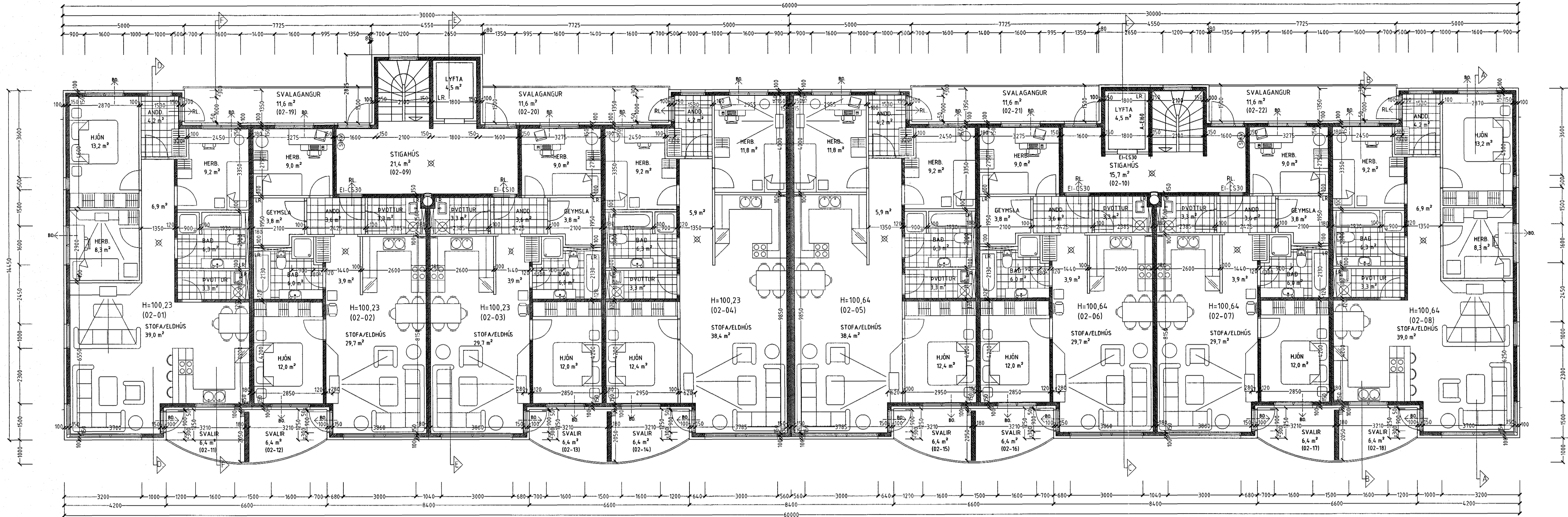
GRUNNMYND 2 HÆÐ. MKV. 1:100.
