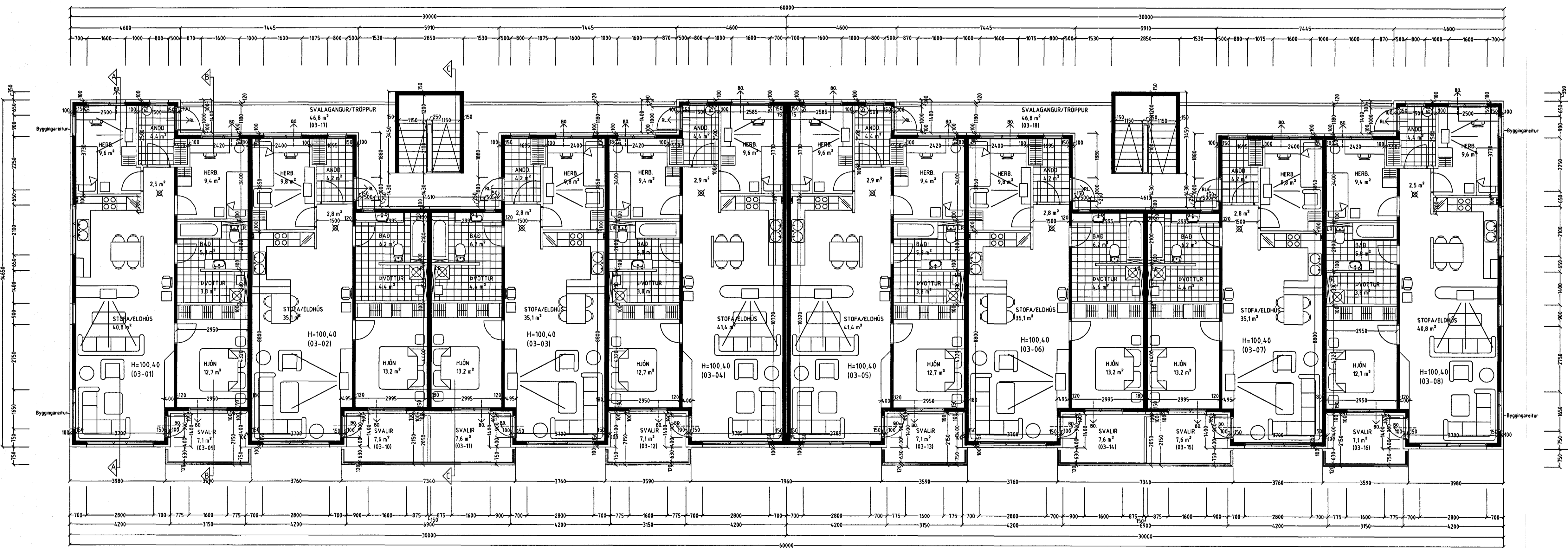
GRUNNMYND 3 HÆÐ. MKV. 1:100.
