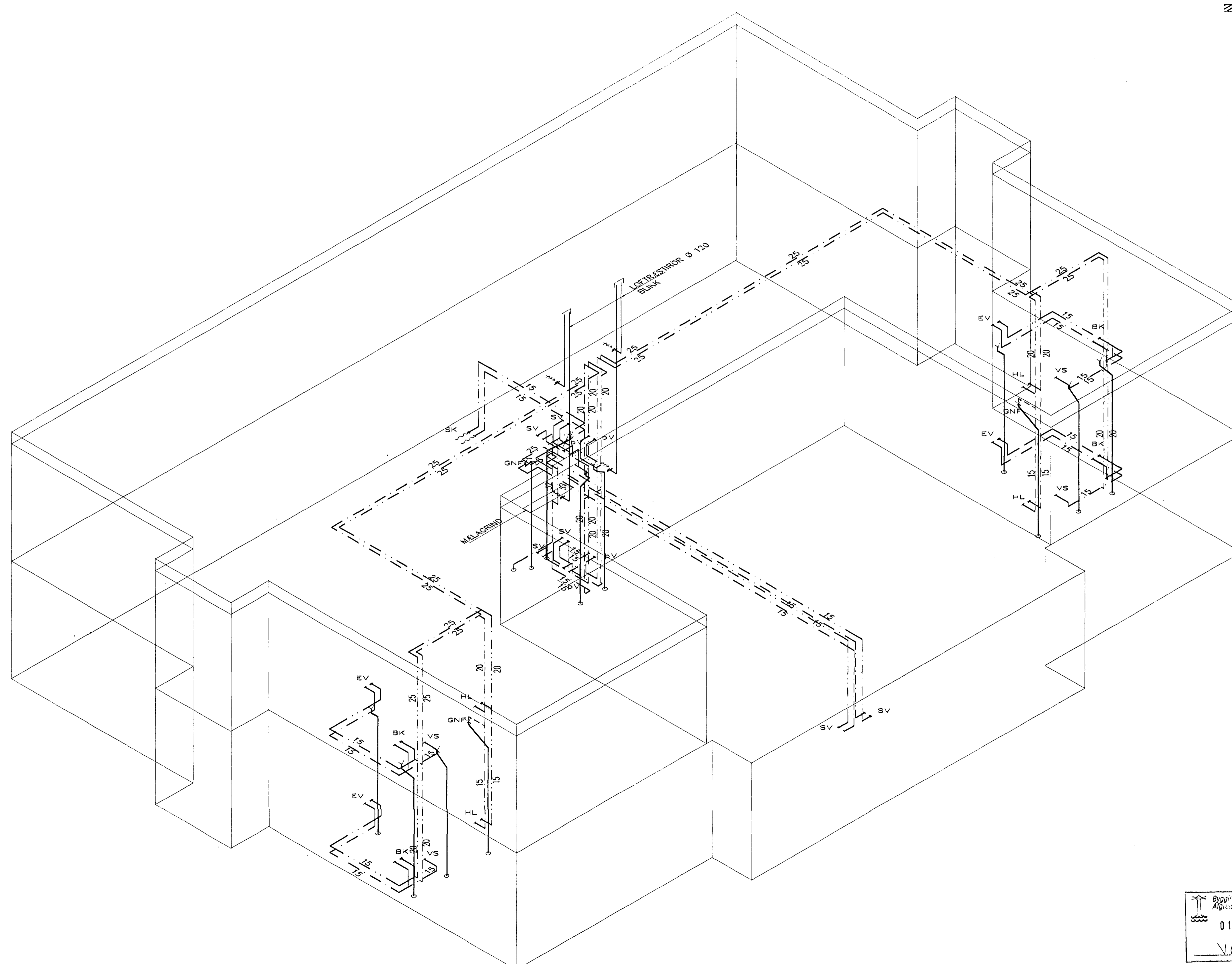
RÚMMYND VATNS OG FRÆRENNSLISLAGNA 1:50
