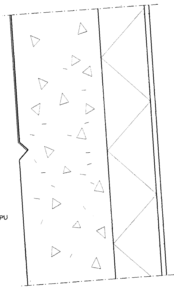
412 SNIÐ Á MÆTINGU SJÓNSTEYPU OG LITAÐRAR PÚSSNINGAR
