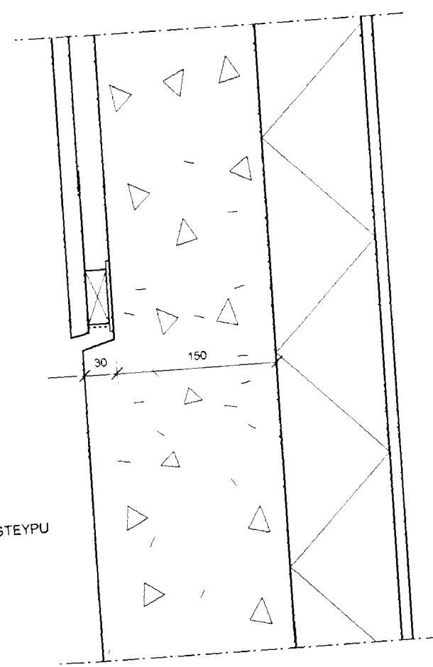
413 SNIÐ Á MÆTINGU SJÓNSTEYPU OG TIMBURKLÆDNINGAR
