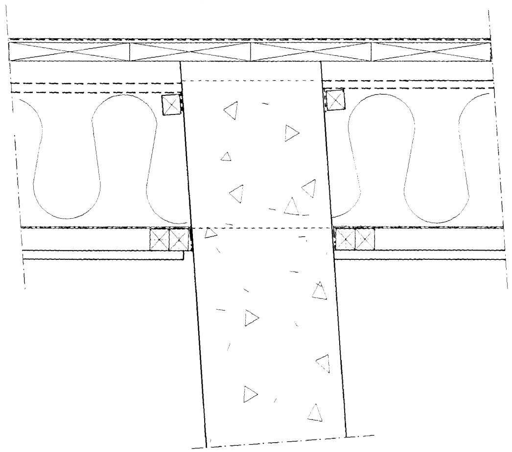
414 REI60 BRUNAVEGGUR Í BÍLAGEYMSLU
