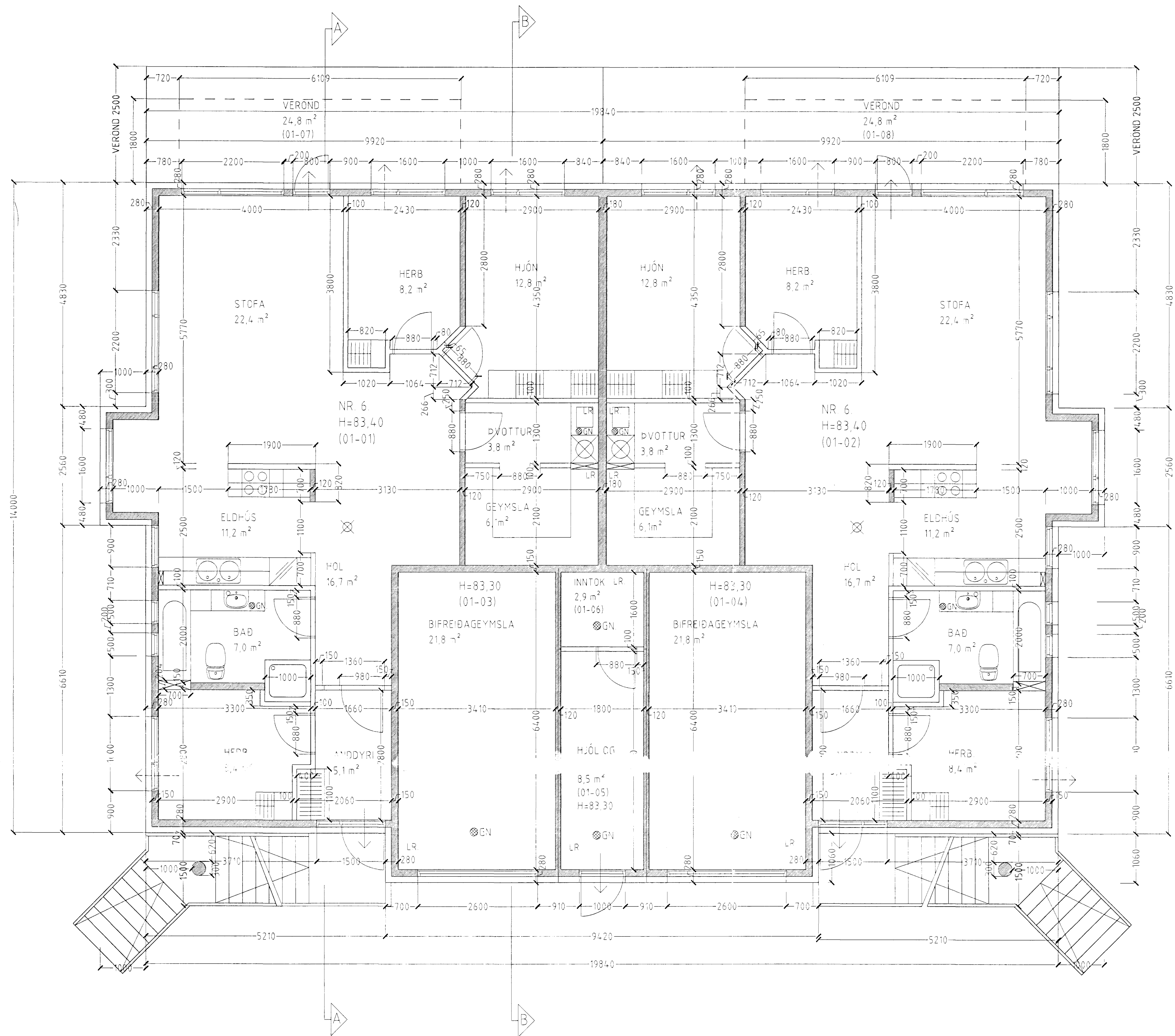
GRUNNMYND 1 HÆÐ MKV. 1:50
