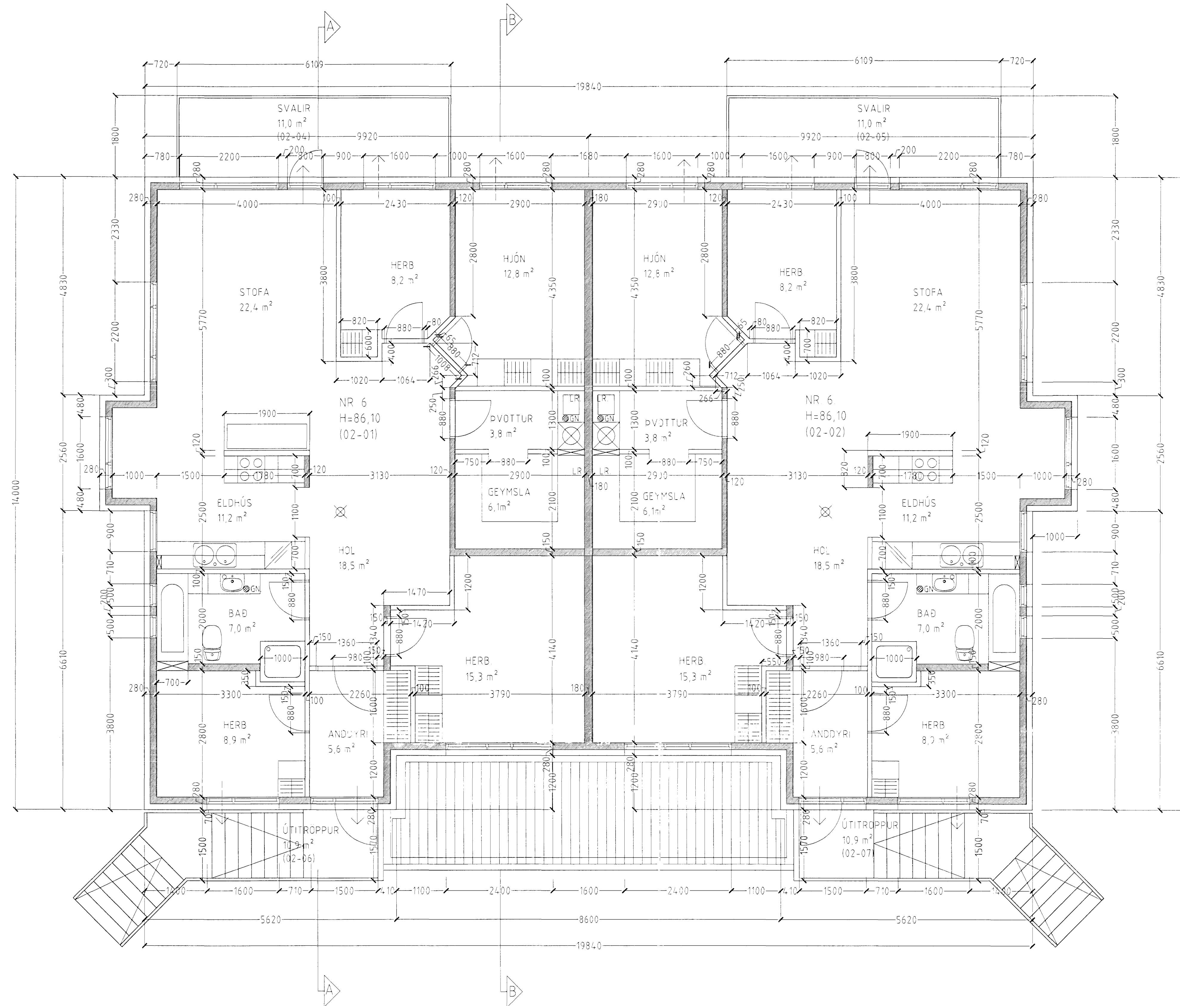
GRUNNMYND 2 HÆÐ MKV. 150.
