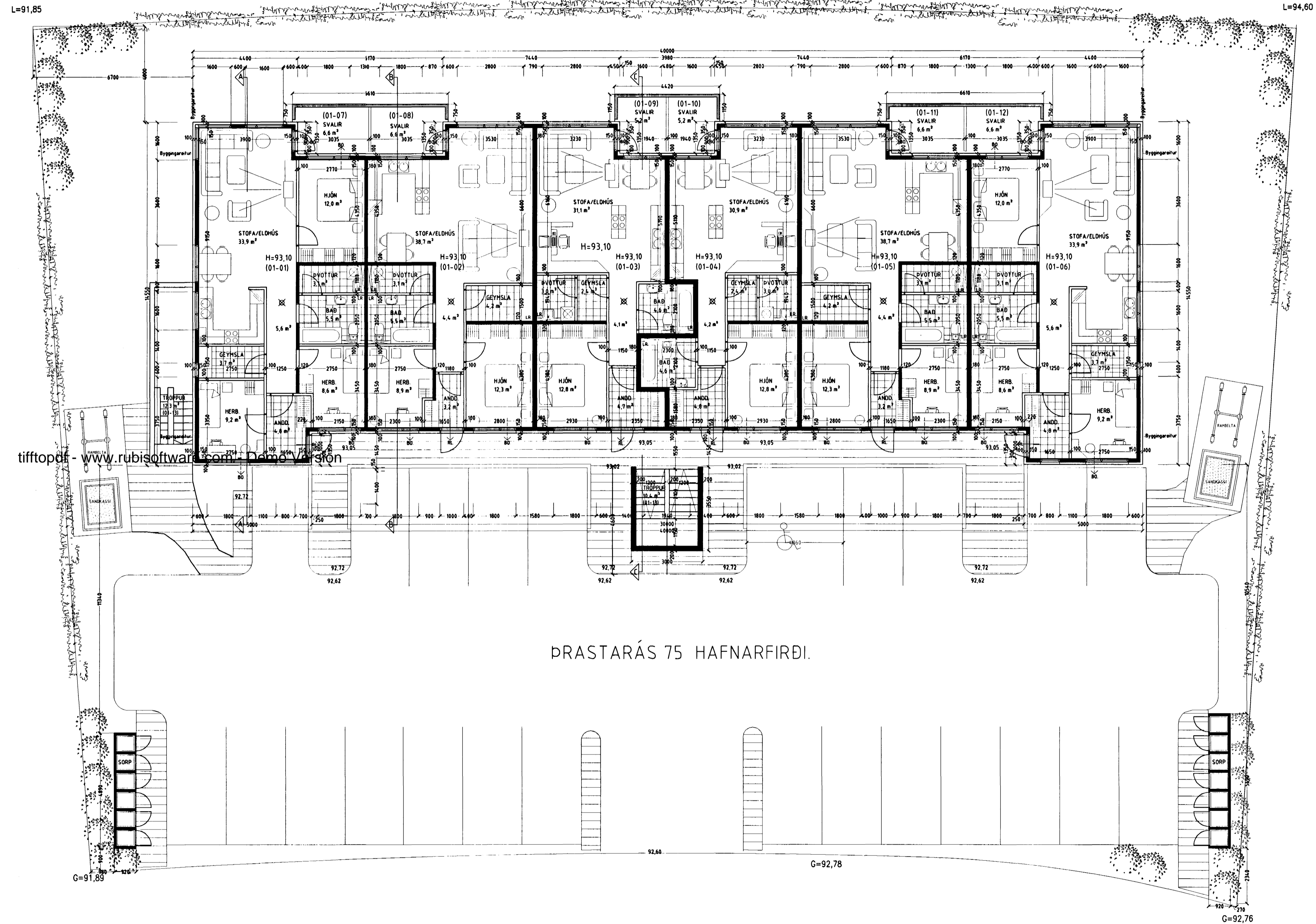
GRUNNMYND 1 HÆÐ MKV 1:100.
